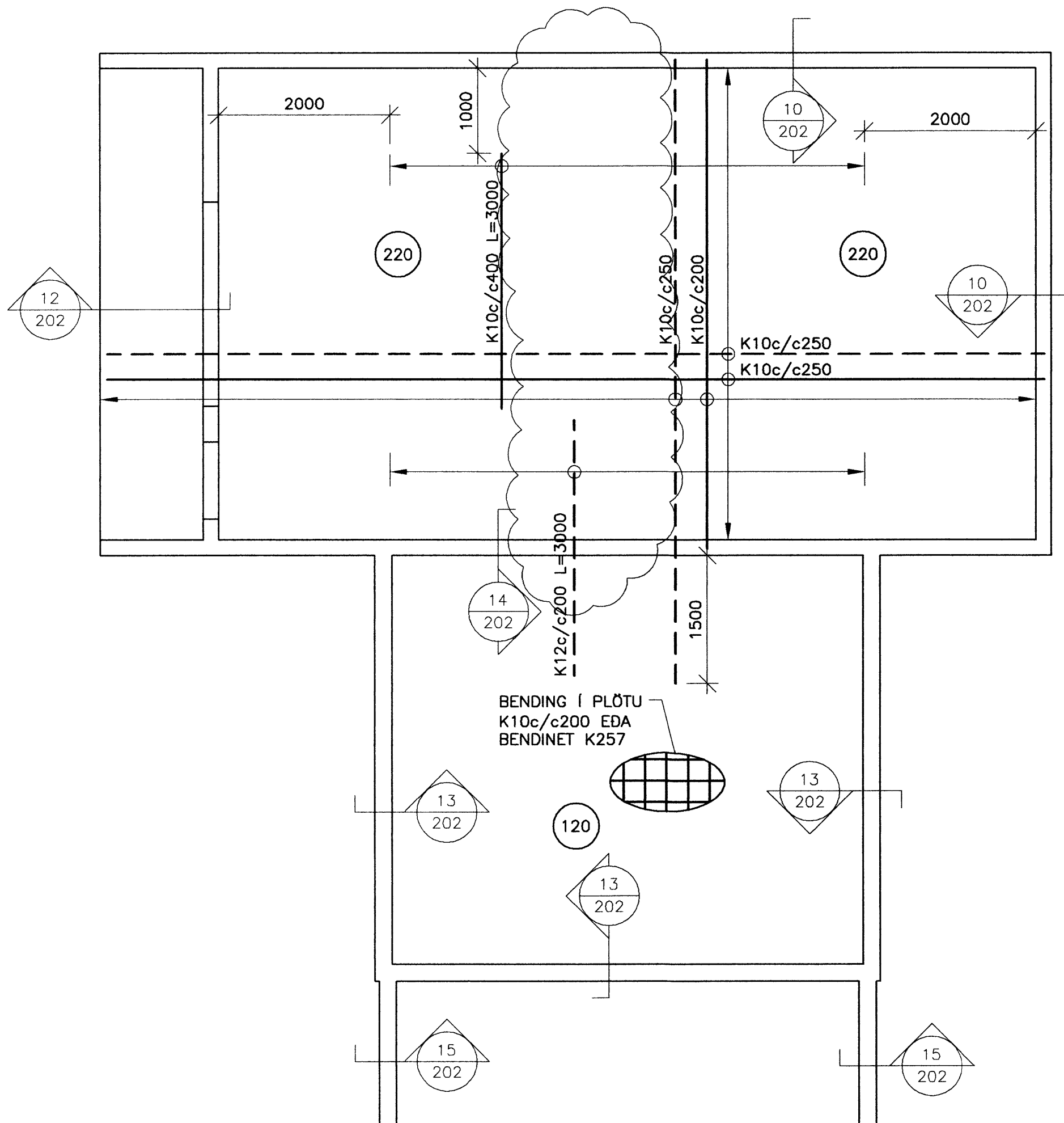
PLATA YFIR KJALLARA. GRUNNMYND. 1:50
