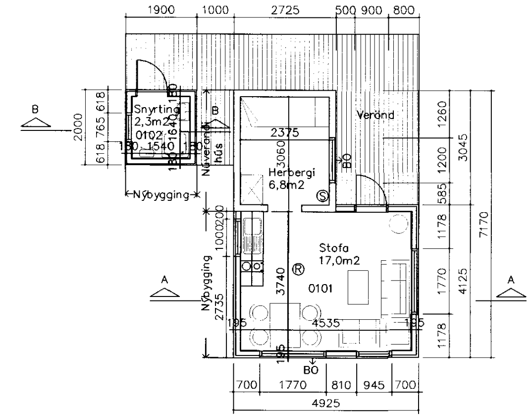
Grunnmynd mkv. 1:100
