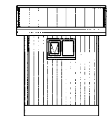
Útlit norður
