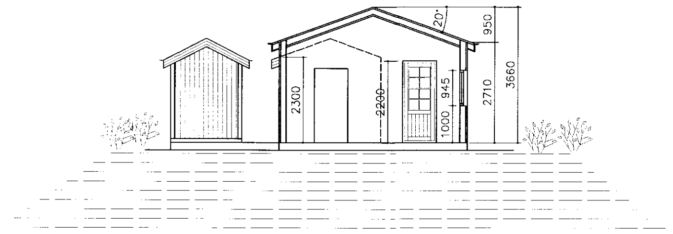
Skurður A-A
