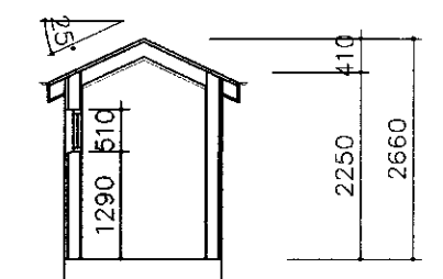
Skurður B-B
