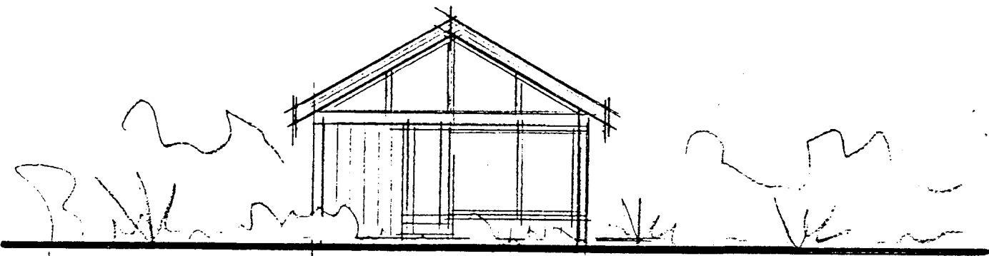
sudlæg átt
