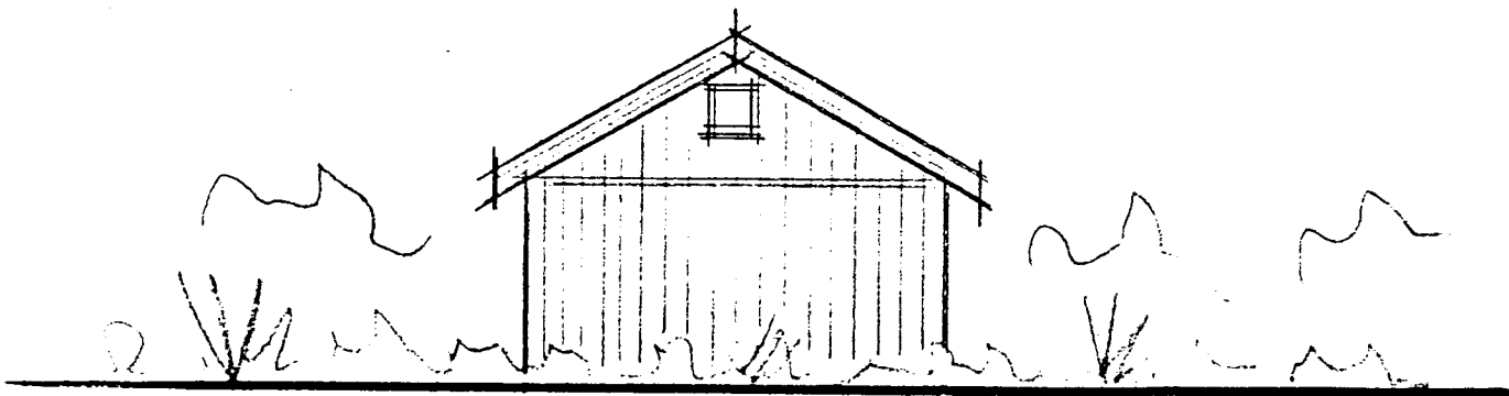
norðlæg átt
