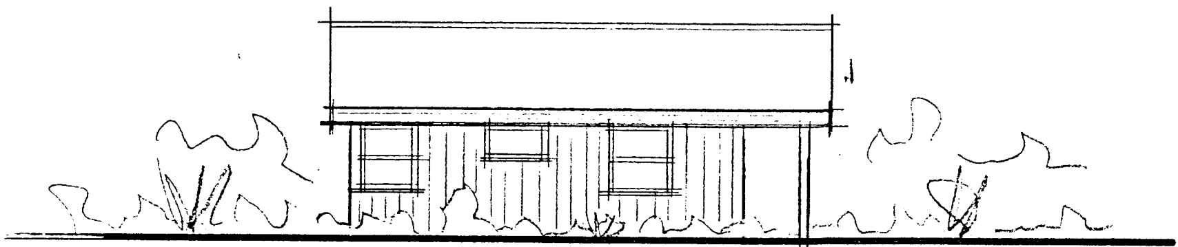
vestlæg átt
