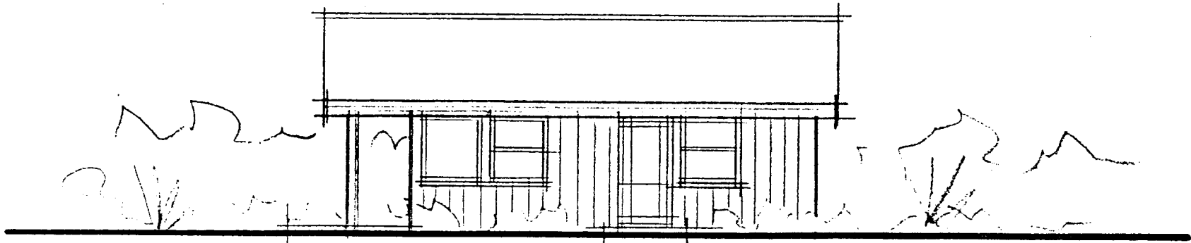
austlæg átt
