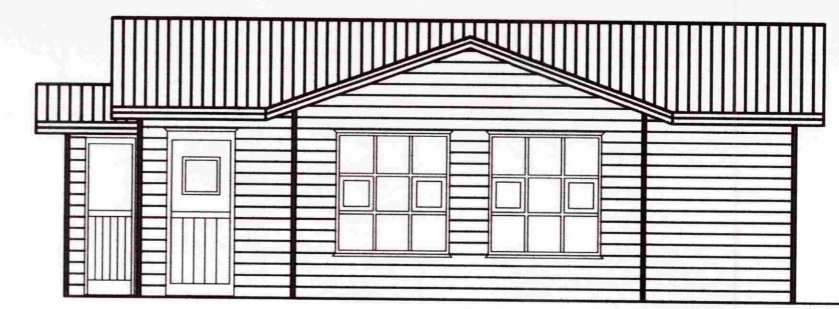
Suður 1:100
