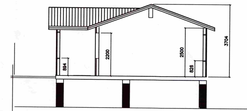
A-A 1:100
