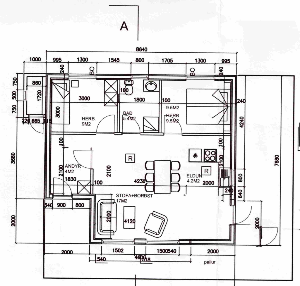
Grundmynd 1:100
