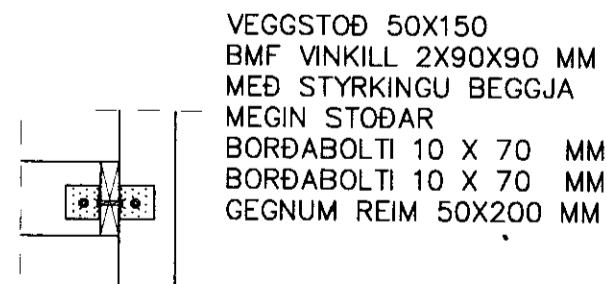
SNID 7 MILLIGÍLF Í MILLIGÓLF
