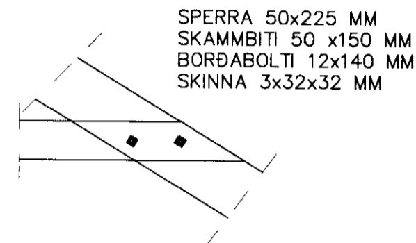
SNID 3 Í SKAMMBITA
