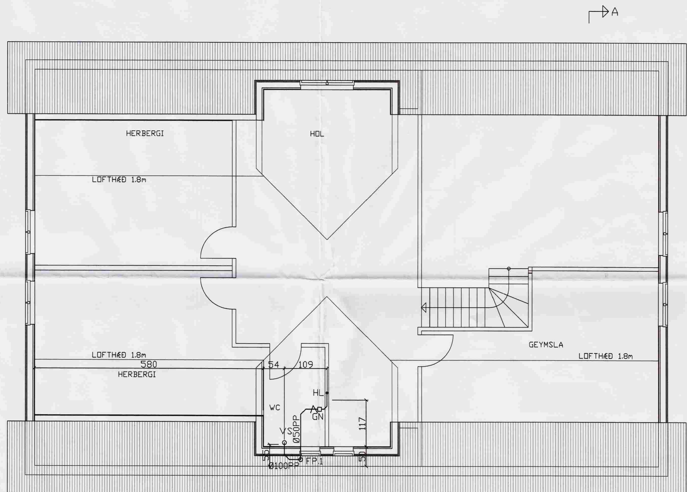
GRUNNMYND 2. HÆÐ
