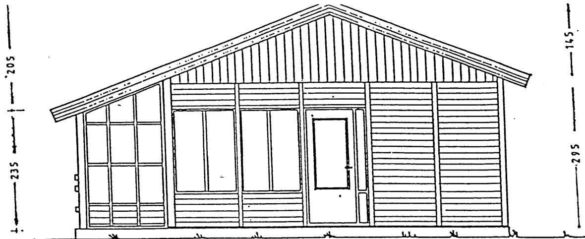
SUDLÆG HLID 1:50
