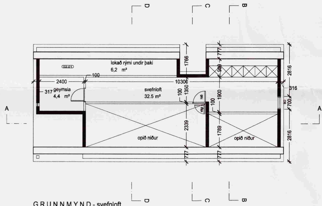
GRUNNMYND - svefnloft
