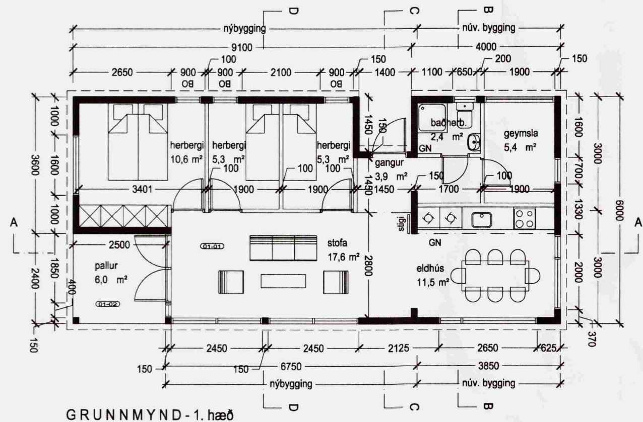
GRUNNMYND - 1. hæð
