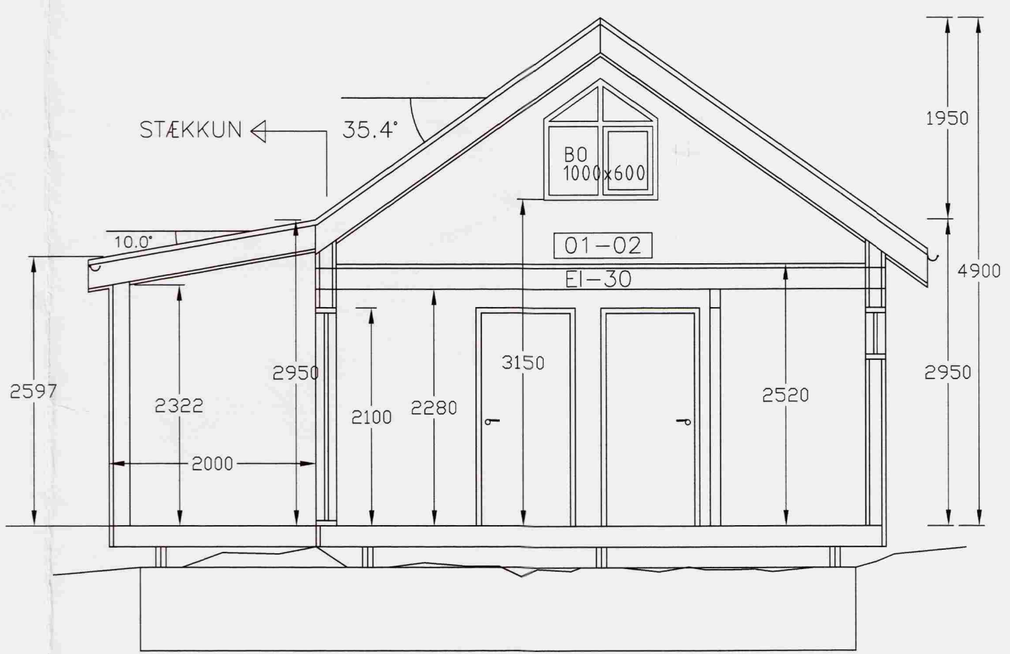
Snið A-A 1:50
