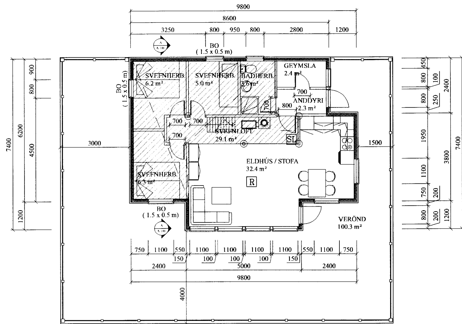
GRUNNMYND 1:100
