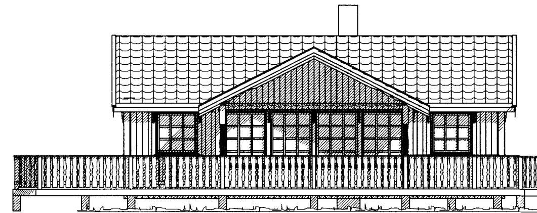
ÚTLIT SUÐUR 1:100
