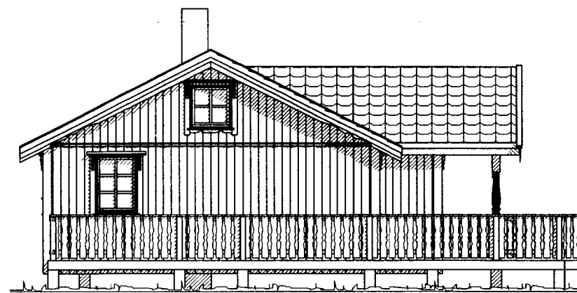
ÚTLIT VESTUR 1:100
