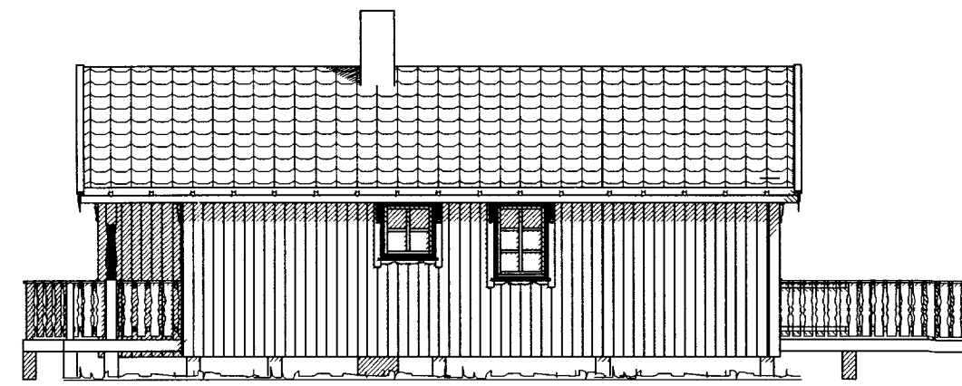
ÚTLIT NORDUR 1:100
