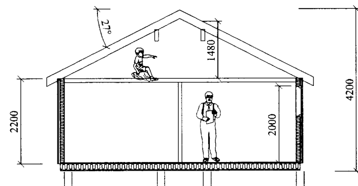
SNEIDING A-A 1:100
