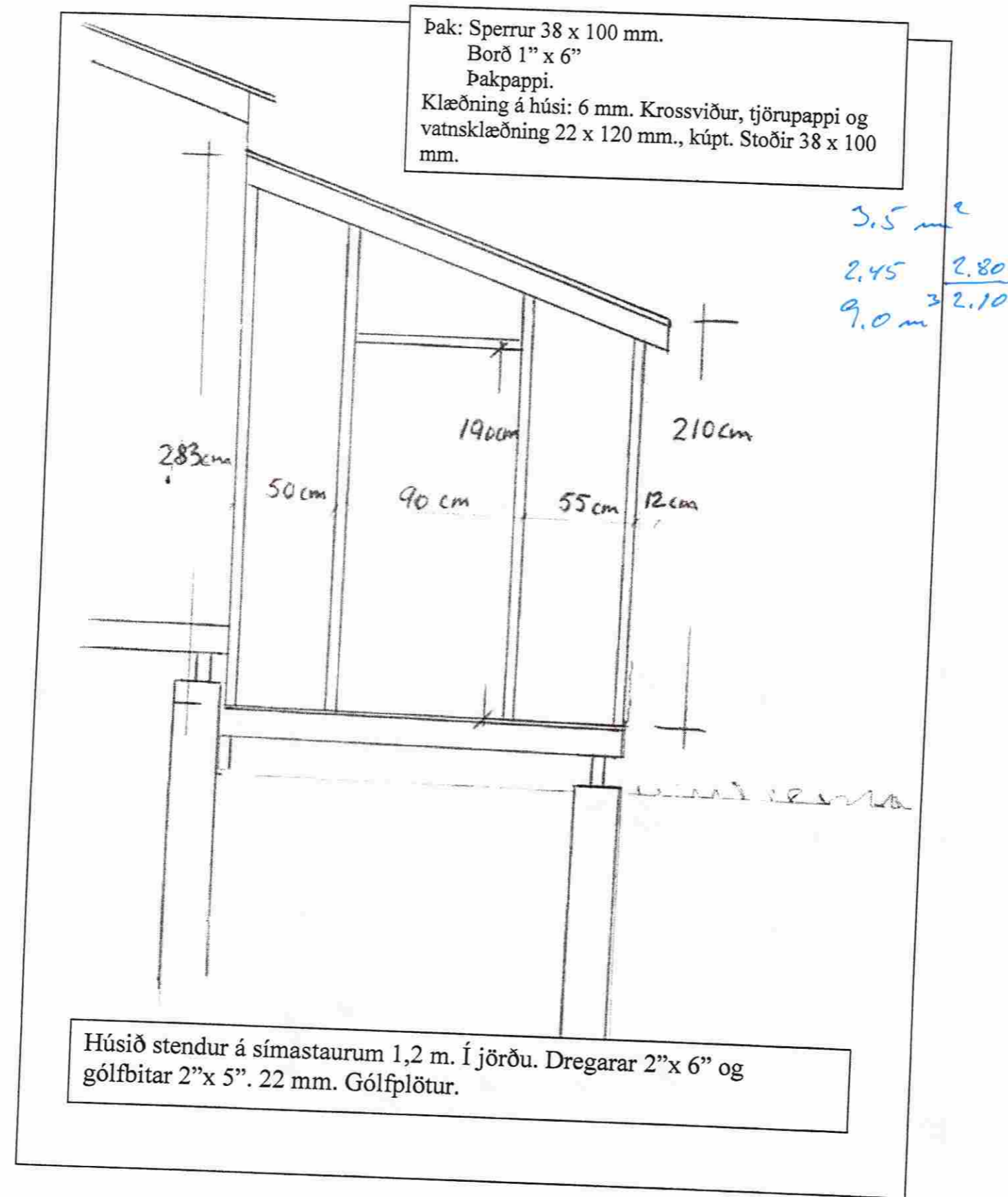
Sumarhús lóð nr. 44 Hallkelshólum Grímsnesi. Geymsla suðurhlið mál 1: 25
