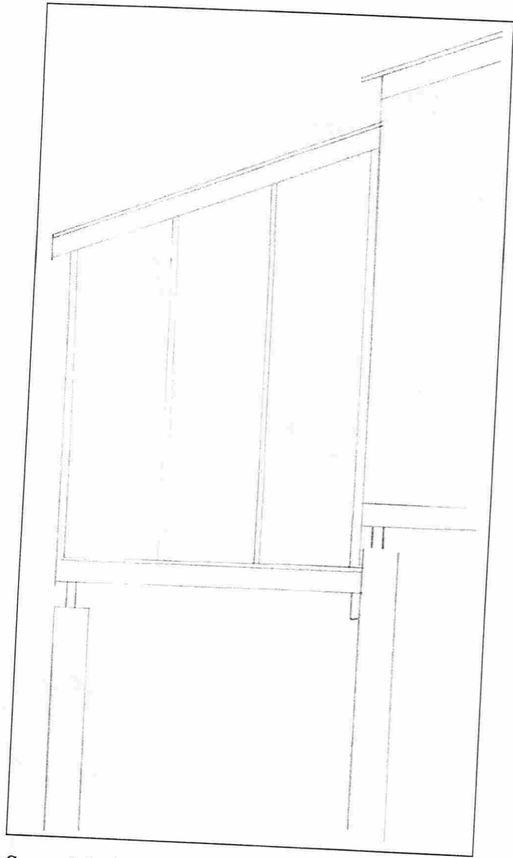
Sumarhús lóð nr. 44 Hallkelshólum Grímsnesi. Geymsla norðurhlið.
