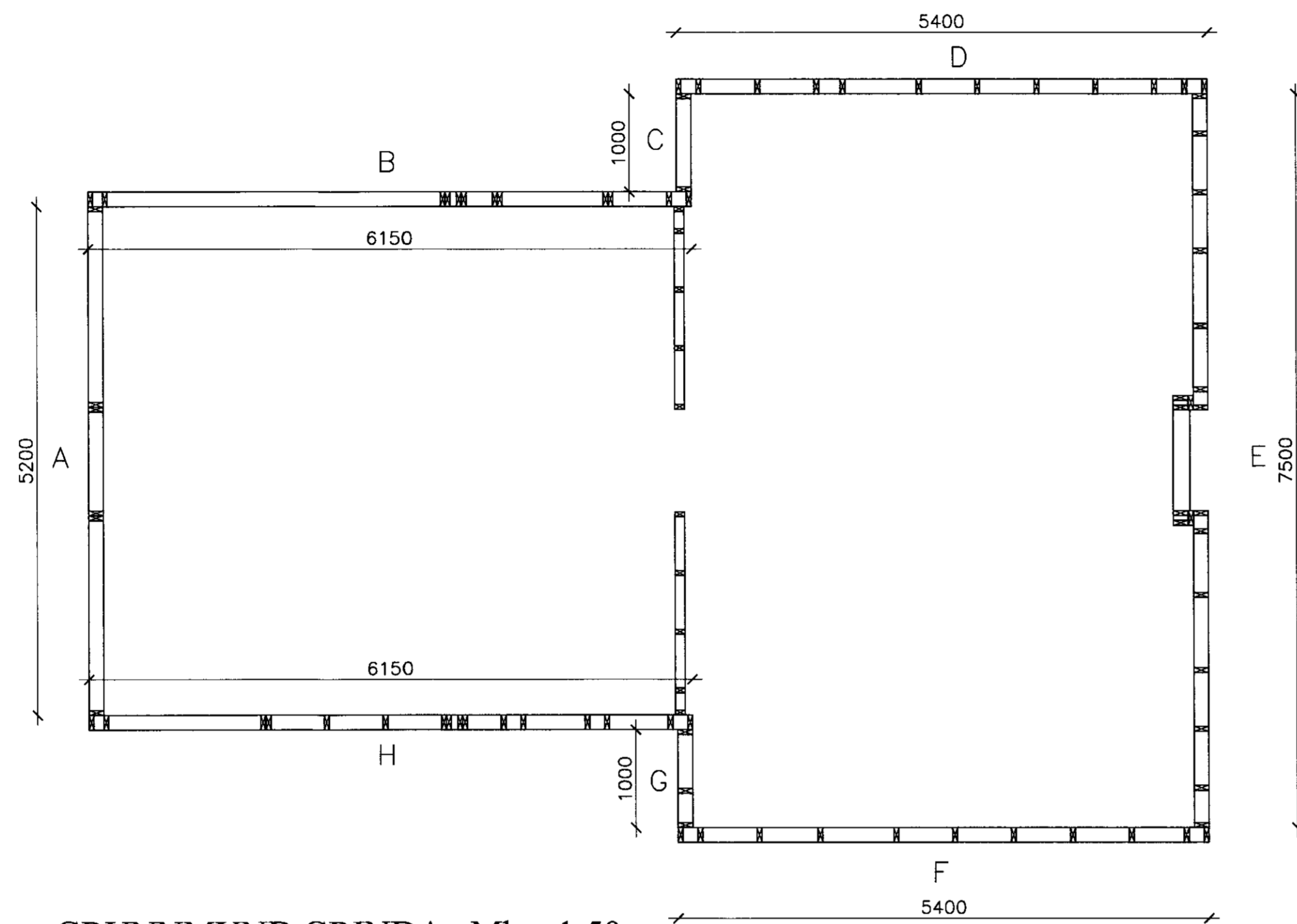
GRUNNMYND GRINDA. Mkv. 1:50
