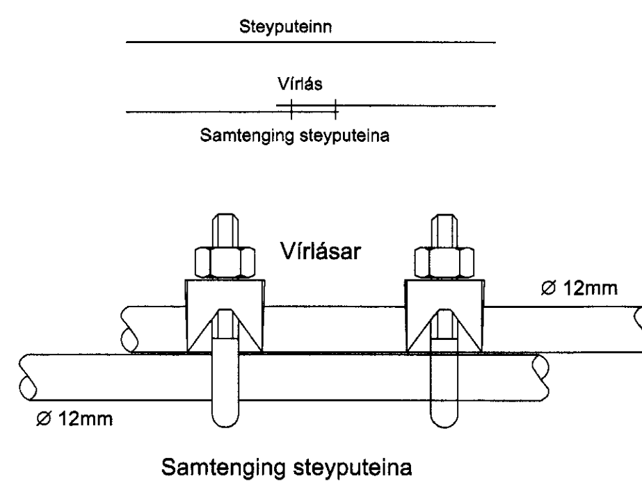
Samtenging steyputeina Setja skal tvo virflása á hver samskeyti
