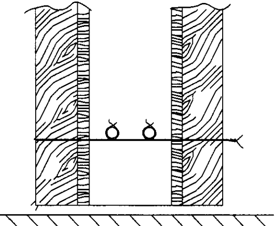
Snið í sökkulvegg Sýnd eru 2 neðstu steypu- styrktarjárn í steypumót ofan á neðstu mótavirum.
