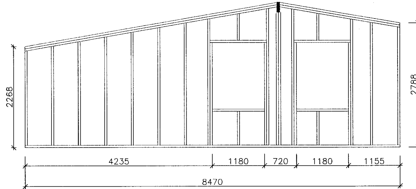
7 Snið 1:50
