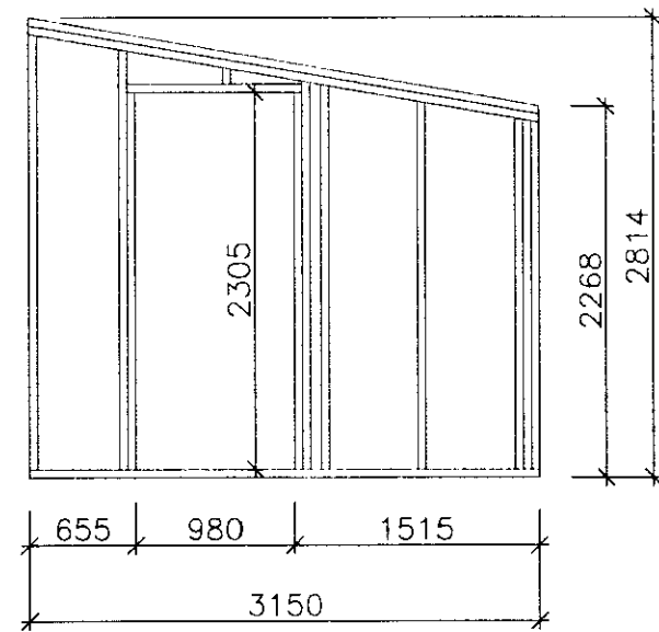
5 Snið 1:50
