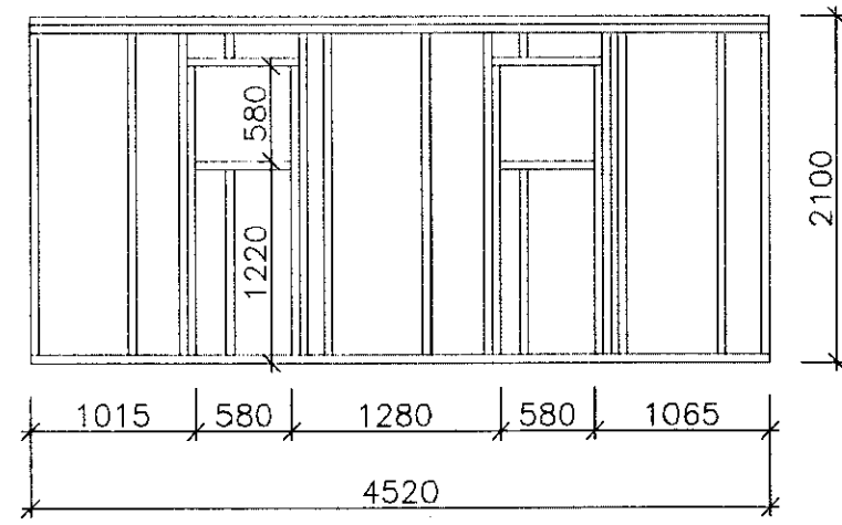
6 Snið 1:50
