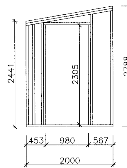
10 Snið 1:50
