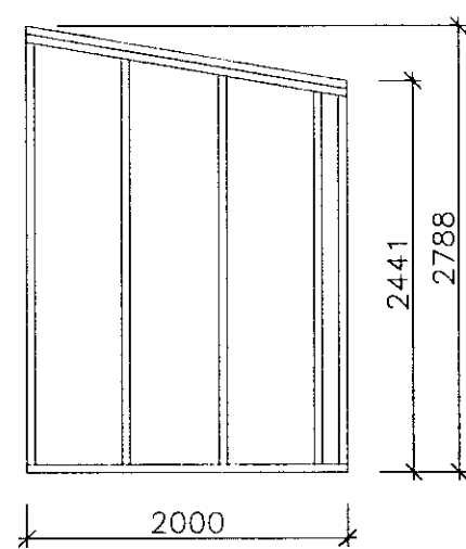
8 Snið 1:50
