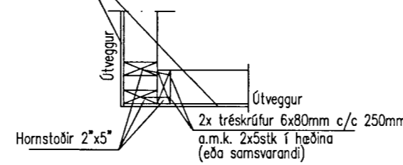
Snið B3 1:20 Almennt lárétt snið í úthorn
