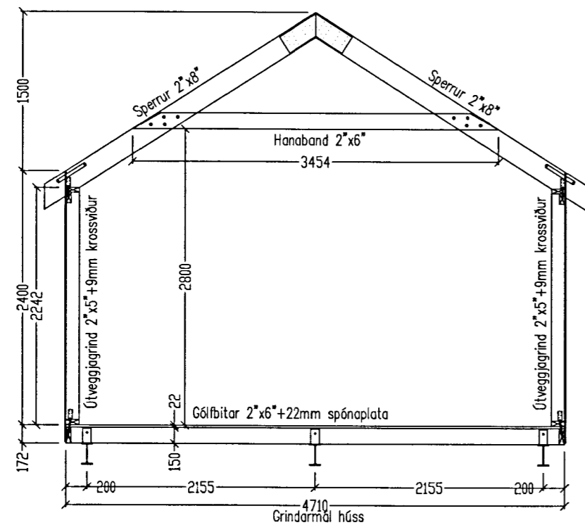
Skurður 1:50
