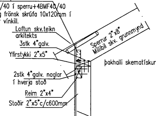
Heiklaða skal útveggjagrind, upp að þakkleðningu (upp á milli sperra) með 9mm krossvið sem vindstífling+vatsvörn og negla í grind með 2 1/2" galv. c/c 150mm í stoðir, yfir- og undirstykki. Snið B1 1:20 Almennt útvegg
