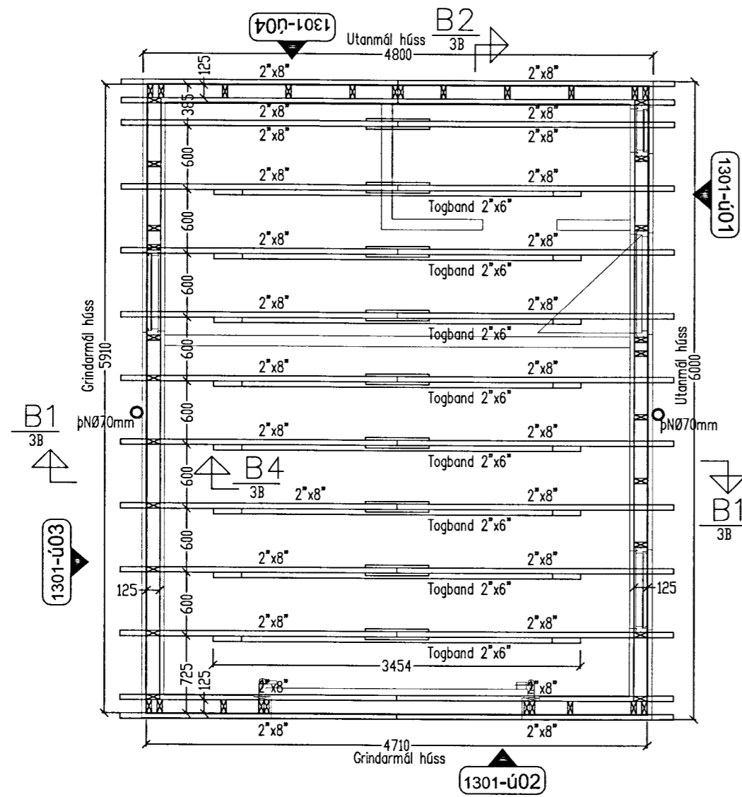
Grunnmynd Þakvirkis 1:50 Tryggja skal loftun framhjá gluggum í útveggjagrind Tryggja skal loftun út um Þakkanta/menisás.
