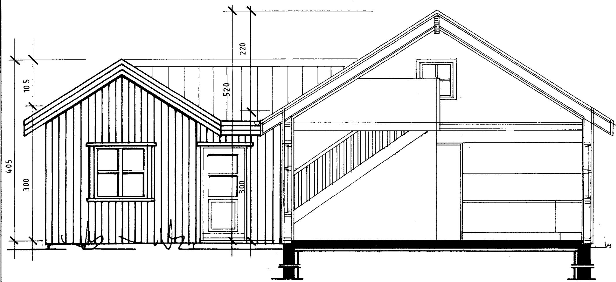
SNIB A-A
