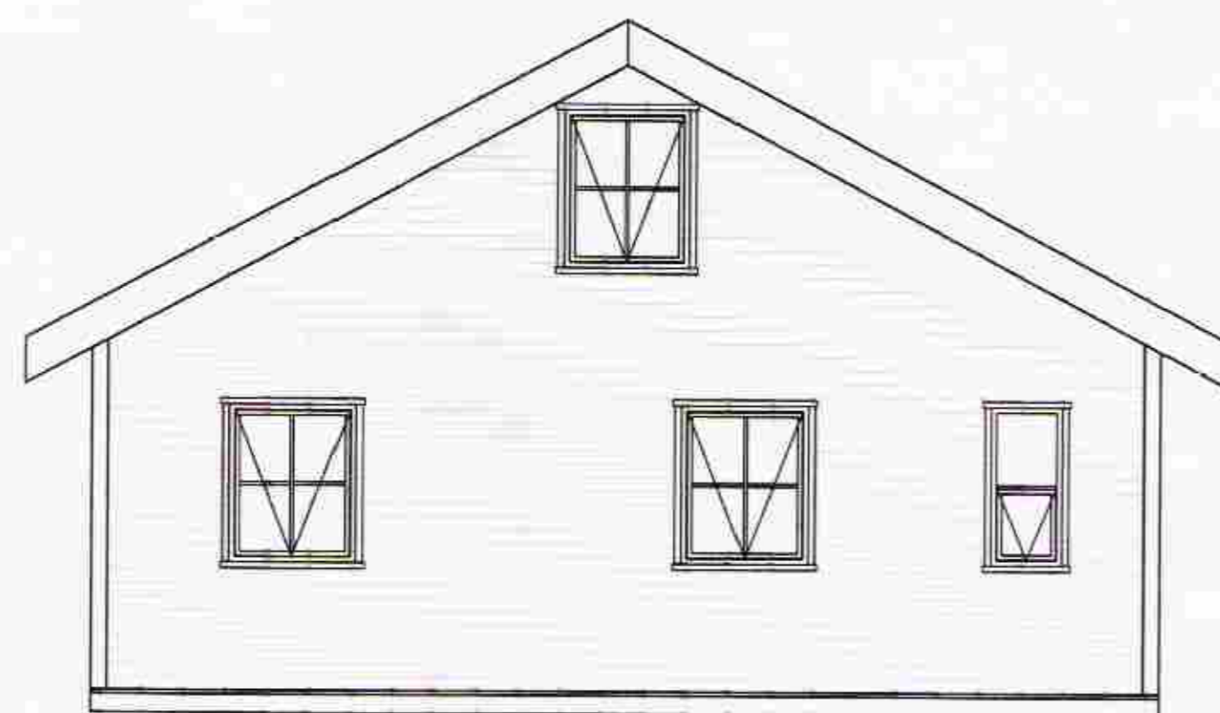
NORÐLÆG HLIÐ
