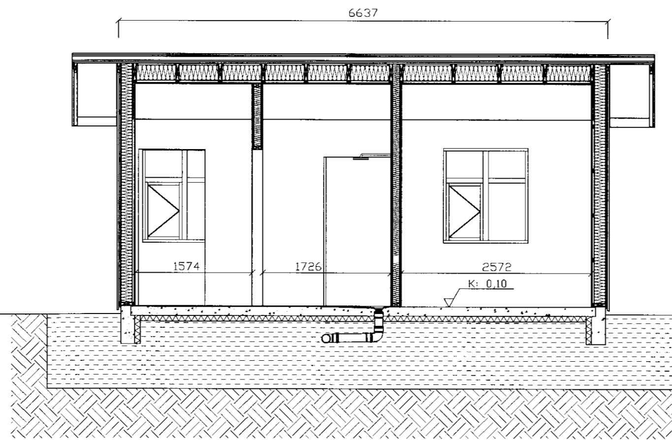
LANGSNIÐ B-B, Mkv. 1:50
