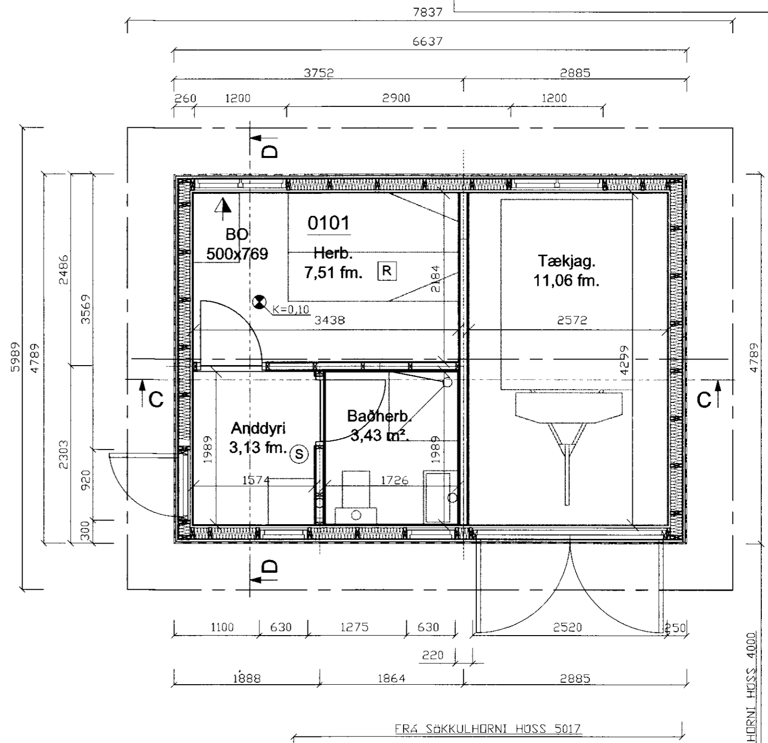
GRUNNMYND, Mkv. 1:50
