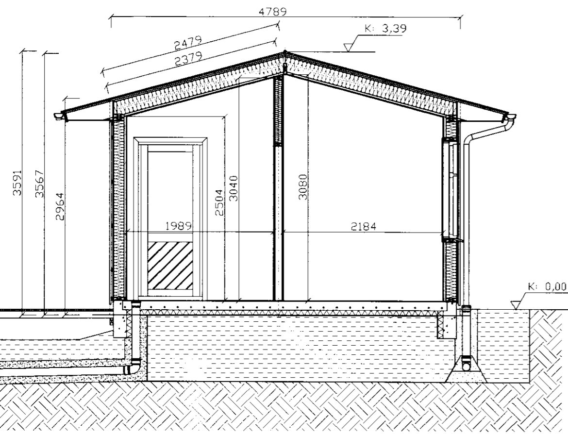
PVERSNIÐ D-D, Mkv. 1:50
