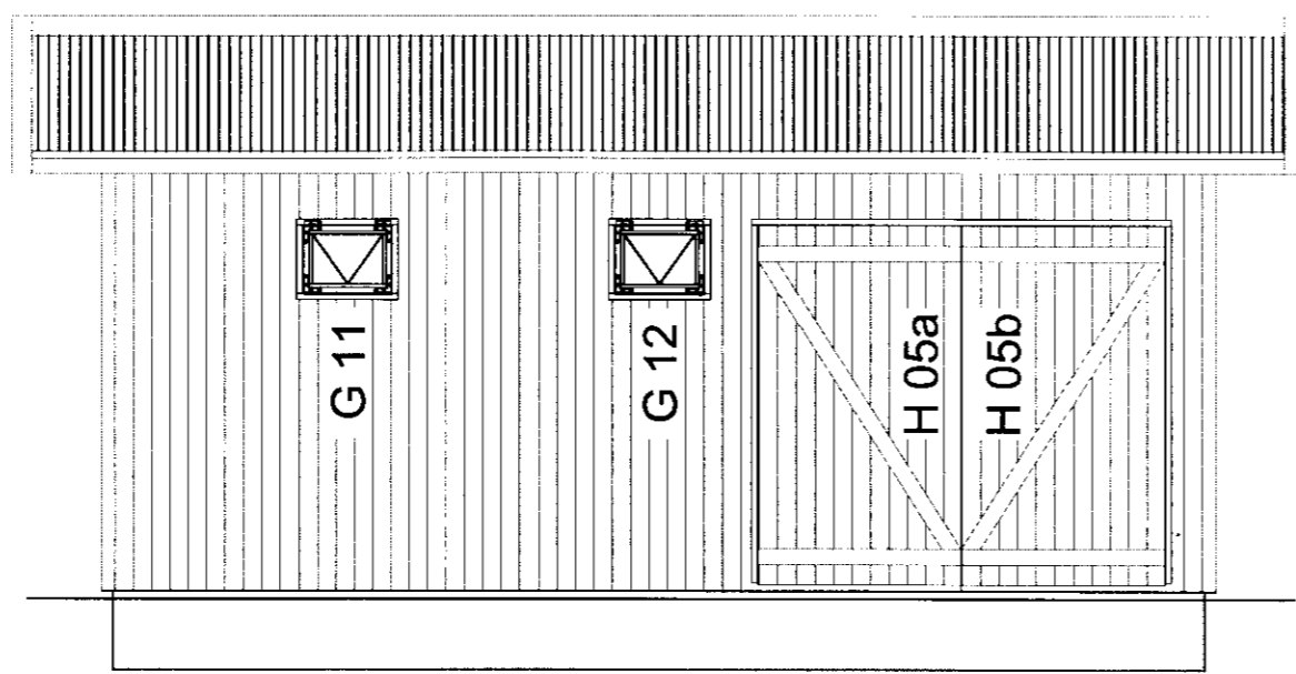
SUÐURHLIÐ. Mkv. 1: 50
