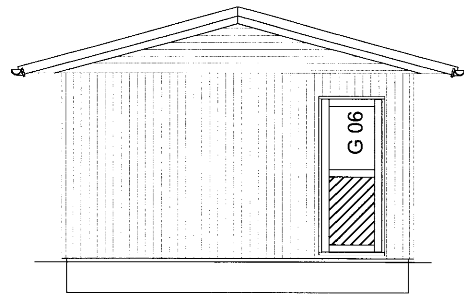
VESTURGAFL. Mkv. 1:50
