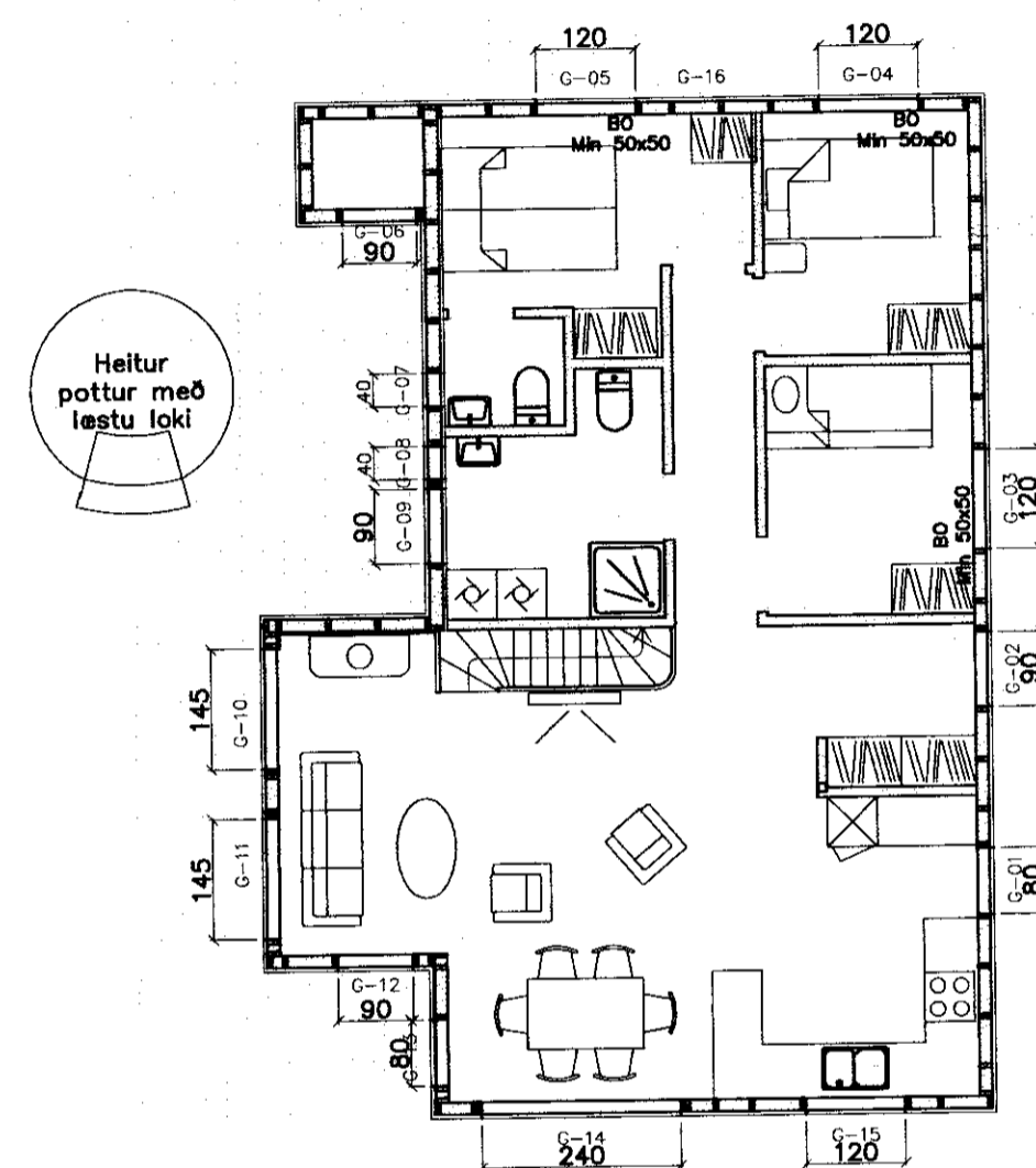
Grunnmynd – Gluggar Mkv. 1:100
