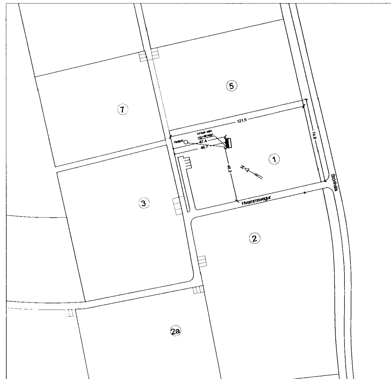
Afstöðumynd 1 : 2000
