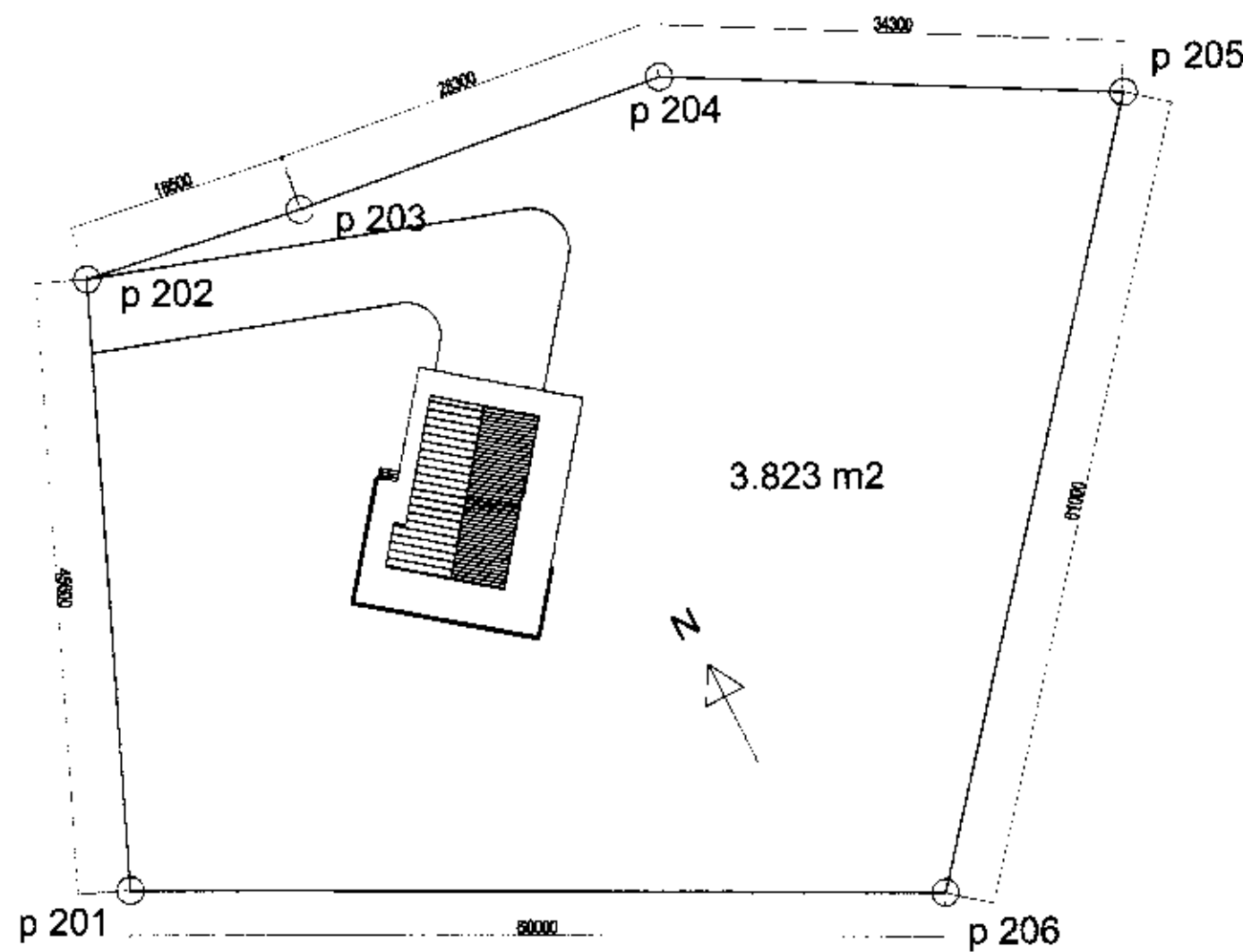
AFSTÖÐUMYND. m: 1/500.
