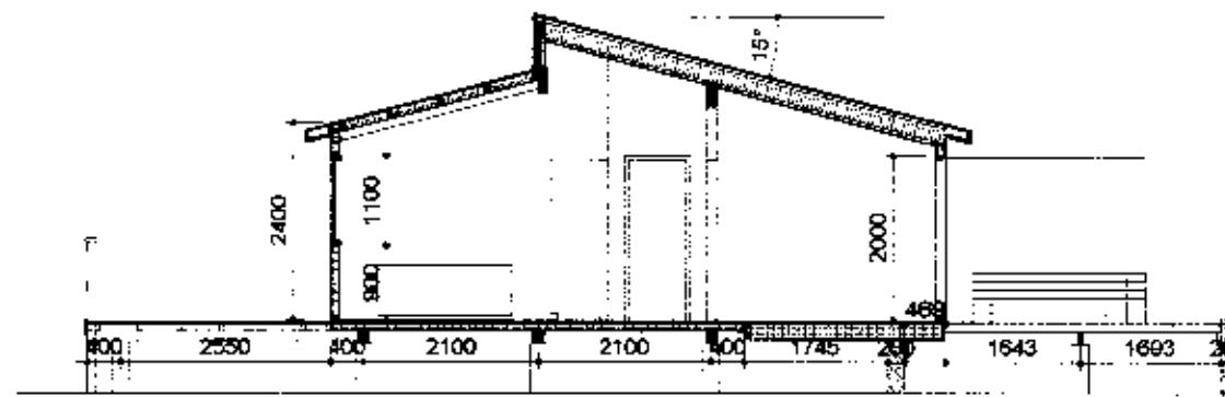
Snið A - A.
