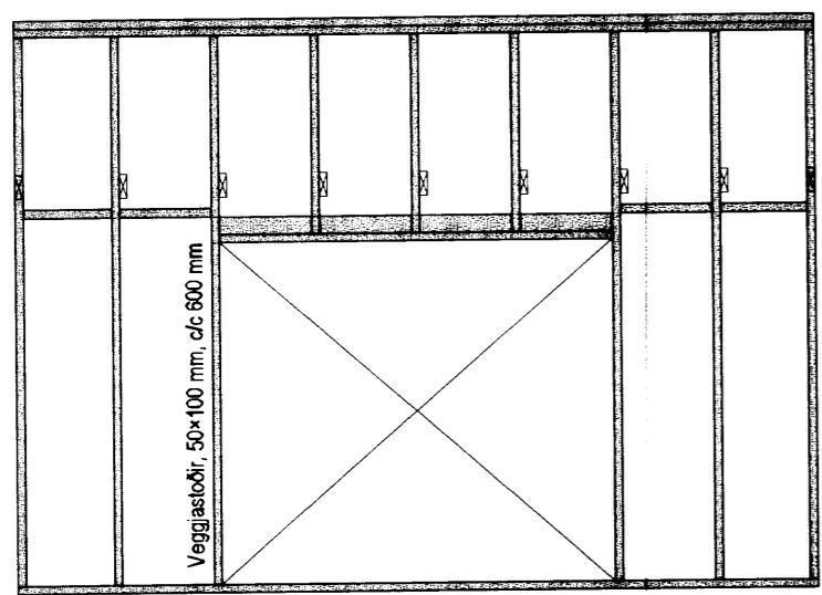
Veggjagrind, norður 1:50
