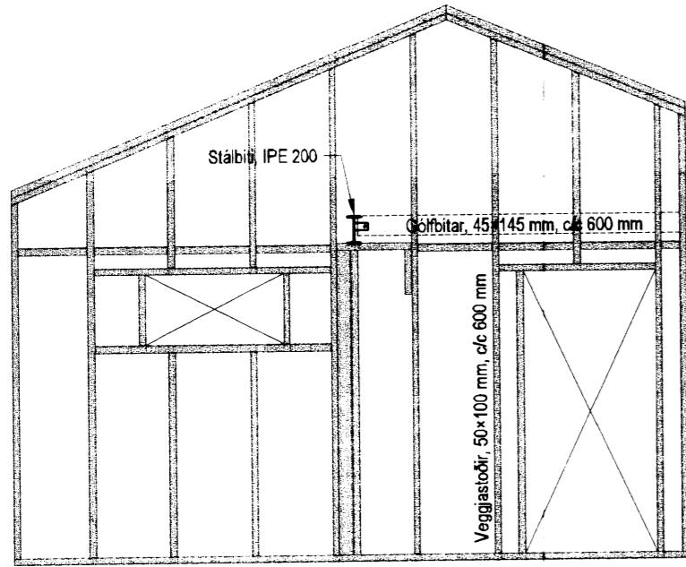
Veggjagrind, austur 1:50
