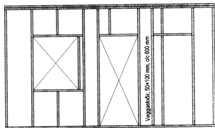
Veggjagrind, suður 1:50
