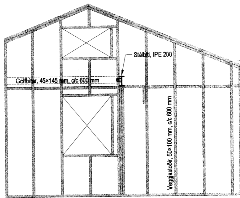
Veggjagrind, vestur 1:50
