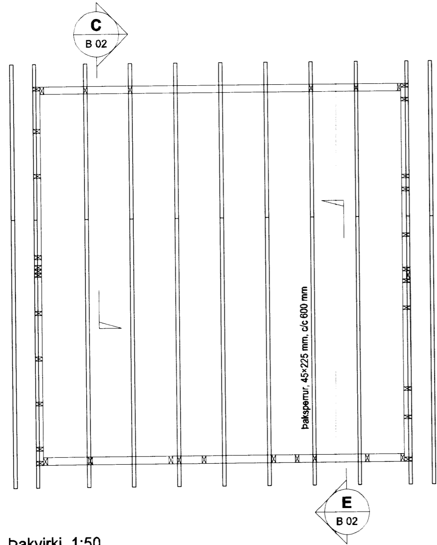
Þakvirki 1:50
