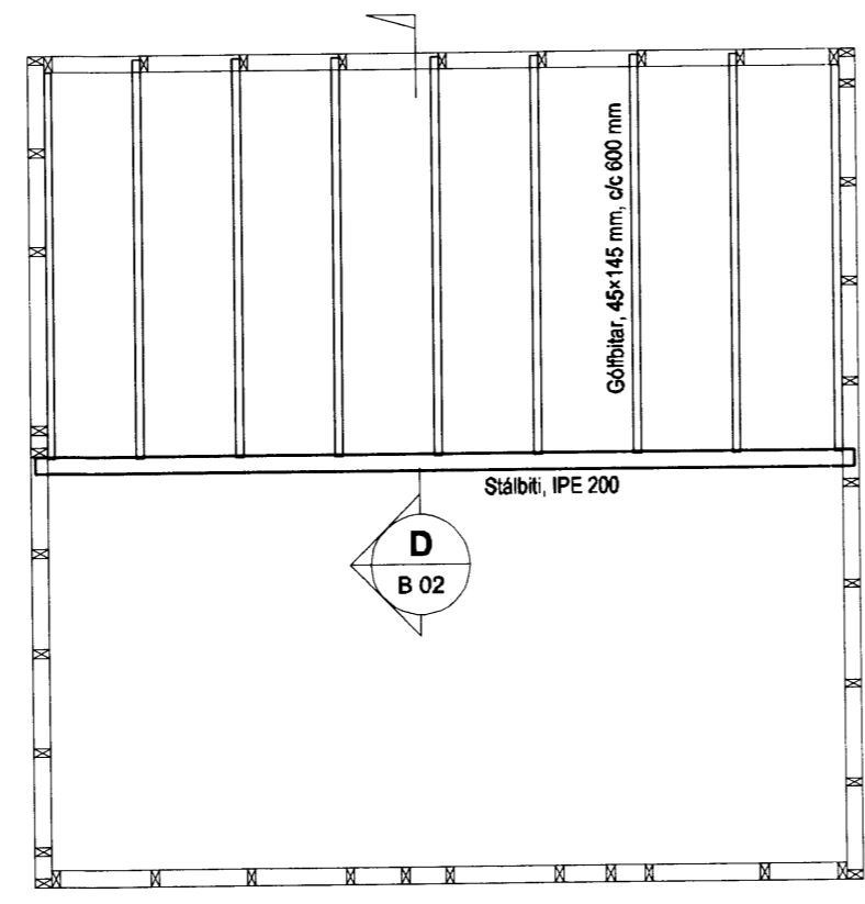
Milligólf 1:50
