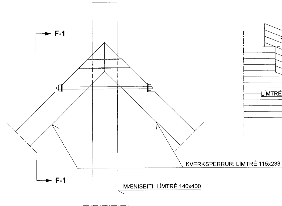
SNID I-I MKV. 1:10
