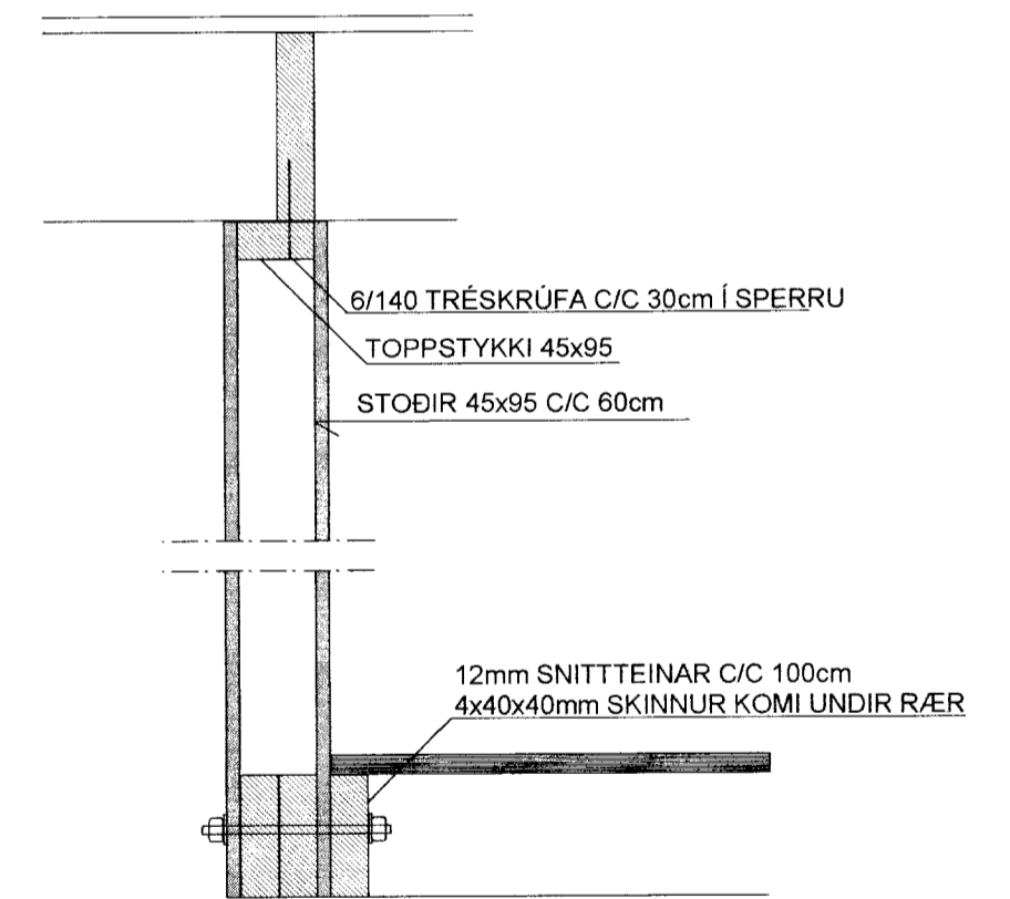
SNID J-J MKV. 1:10
