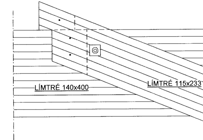
SNID F-1 MKV. 1:10
