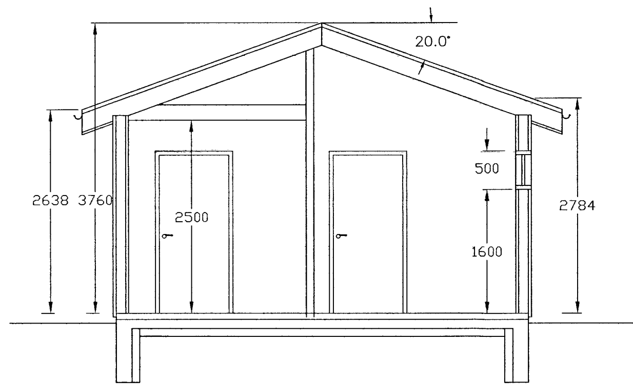
Snið B-B 1:50
