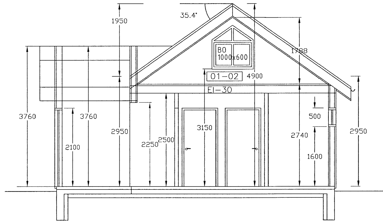
Snið A-A 1:50
