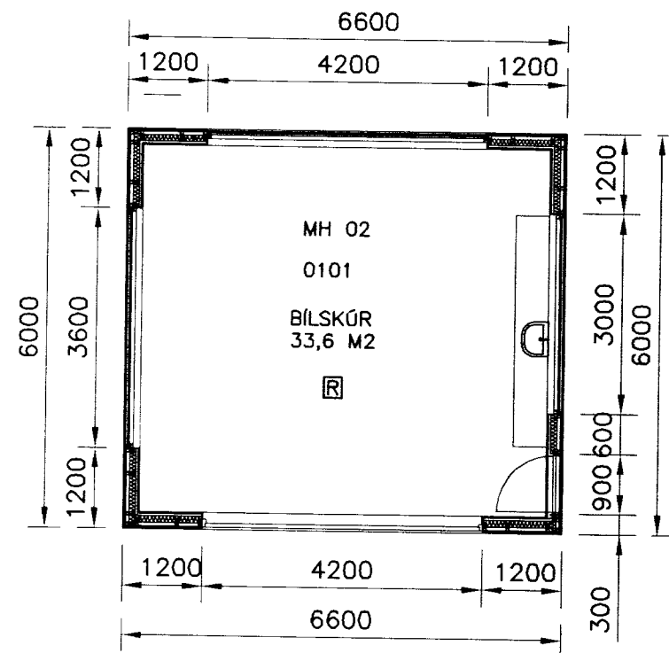
GRUNNMYND 1:100
