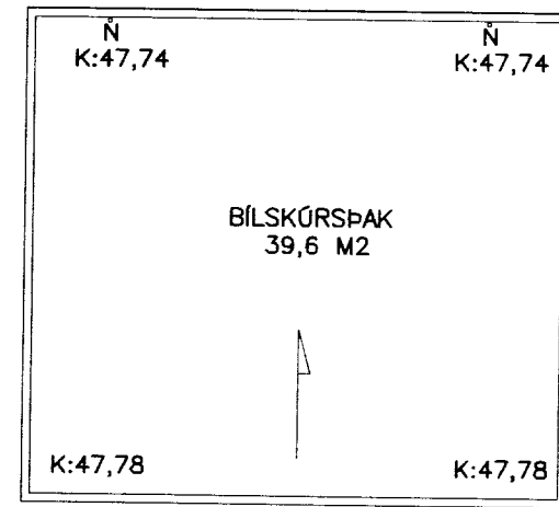
GRUNNMYND, ÞAK 1:100
