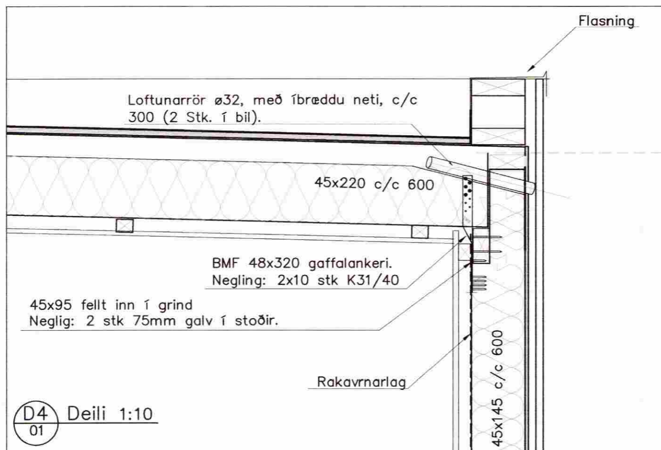
D4a Deili 1:10 01
