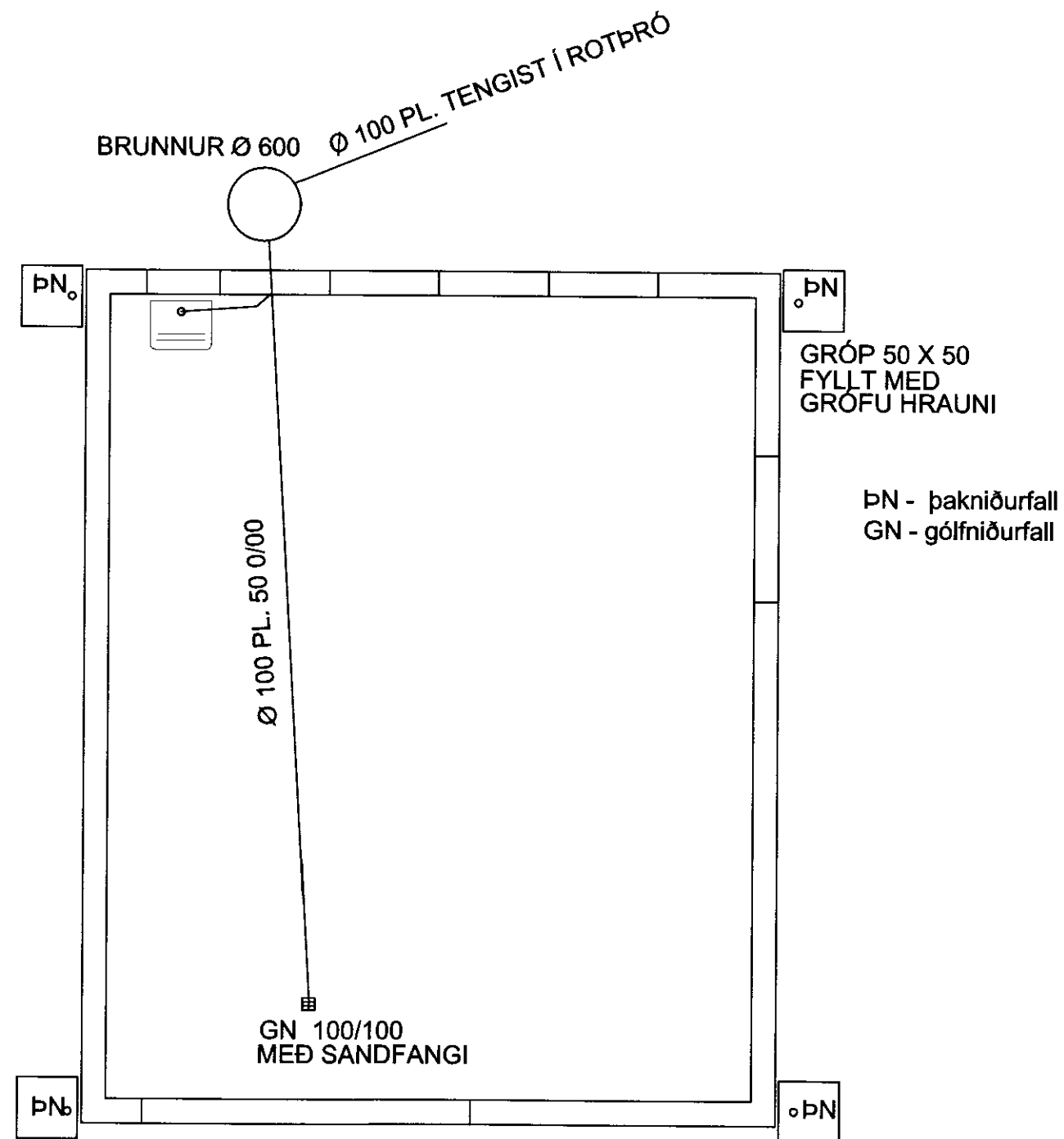
FRÁRENNSLI GRUNNMYND 1:50
