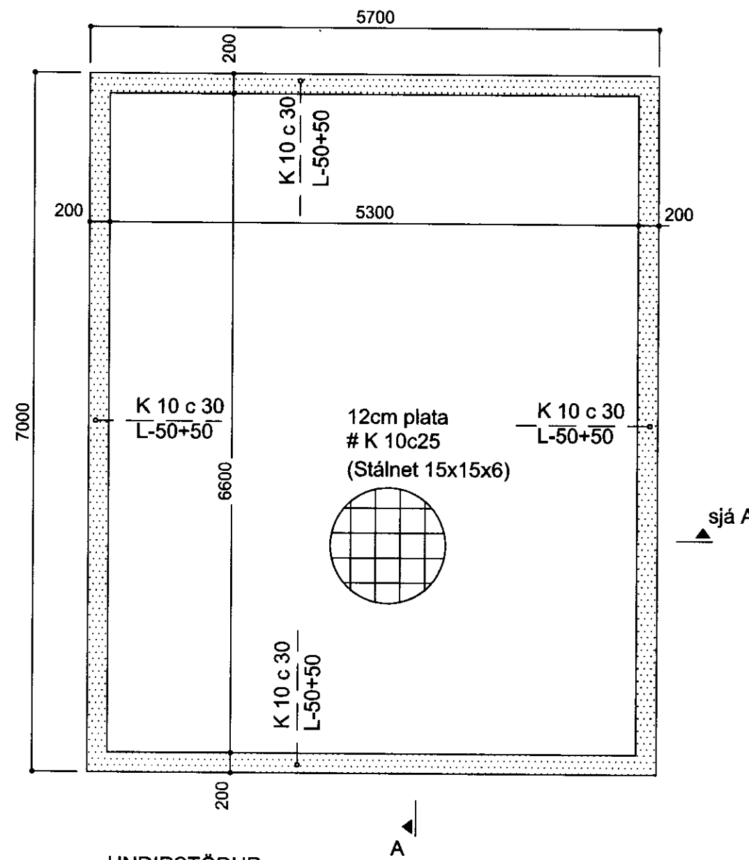
UNDIRSTÖÐUR GRUNNMYND 1:50
