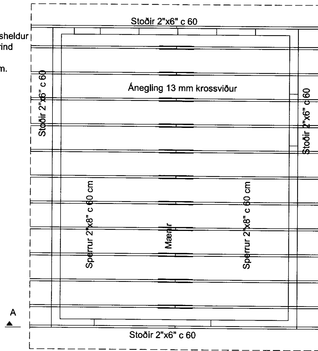
ÞAKBITAR GRUNNMYND 1:50
