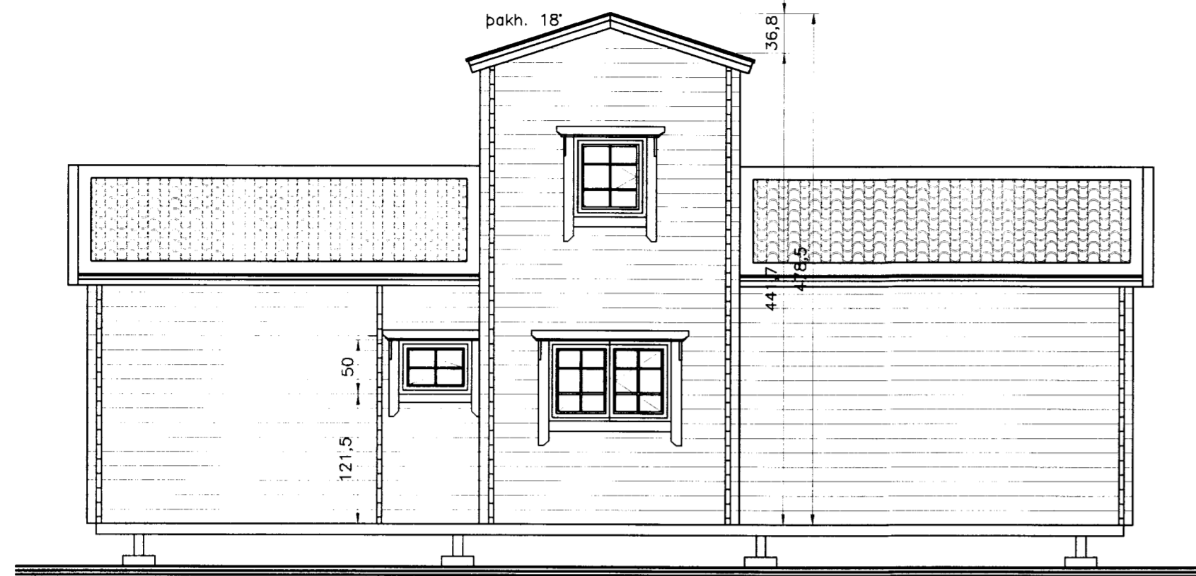
Norðurhlíð 1:50
