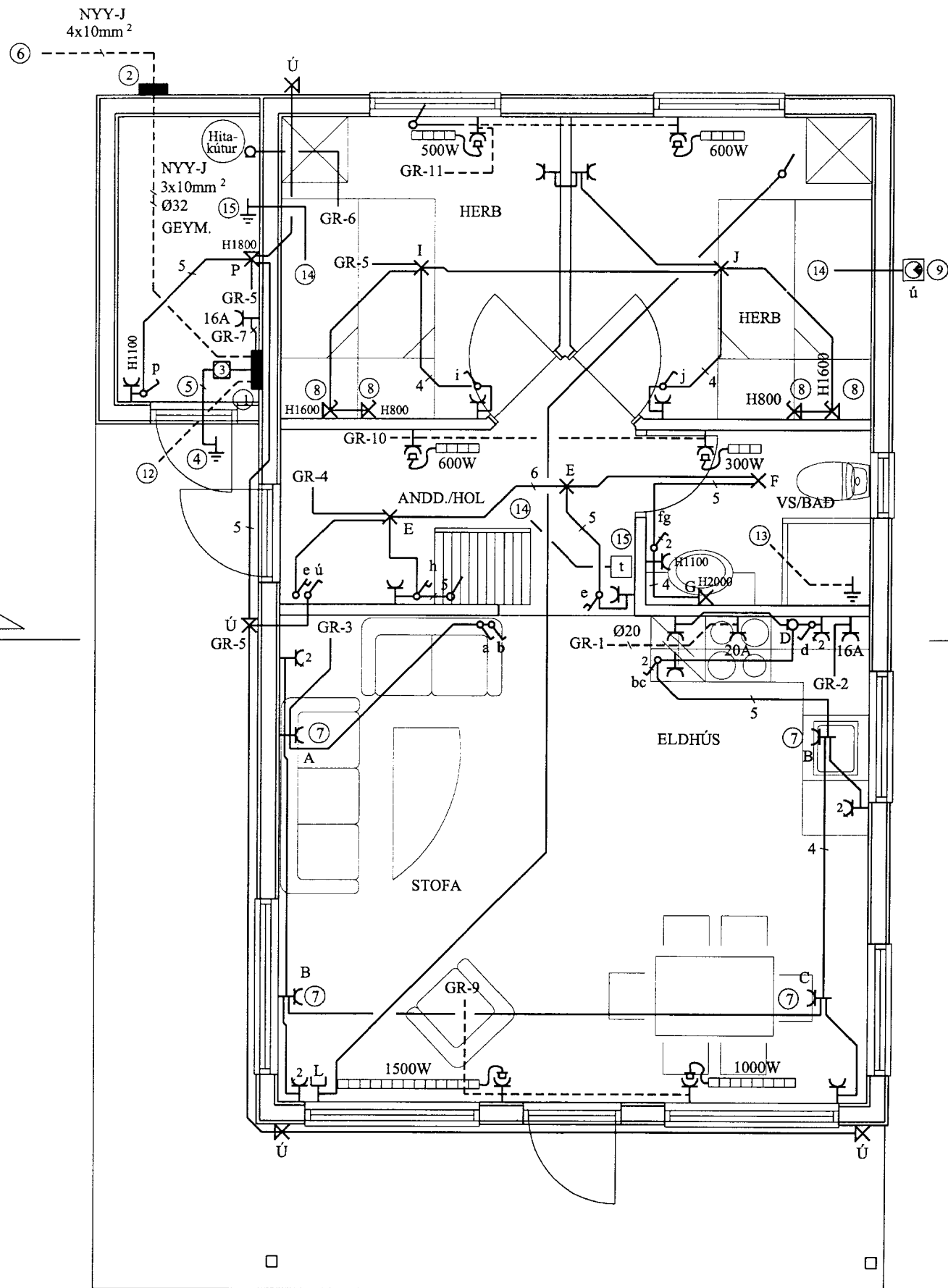
GRUNNMYND JARÐHÆÐ RAFLAGNIR
