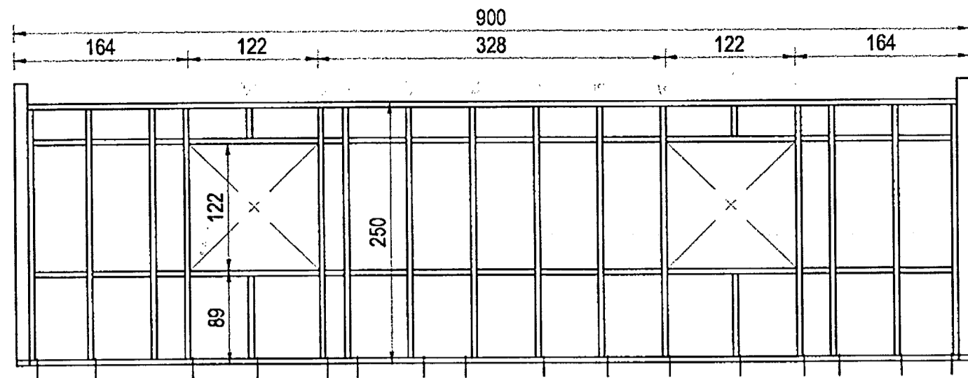
HÚS B, TIMBURGRIND SUÐUR HLIÐAR
