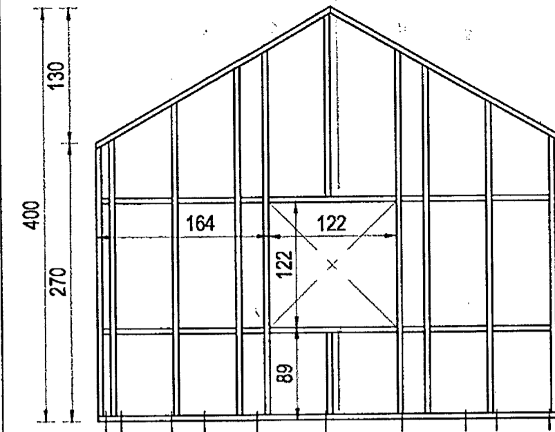
HÚS B, TIMBURGRIND VESTUR HLIÐAR
