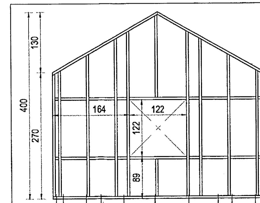
HÚS A, TIMBURGRIND VESTUR HLIÐAR
