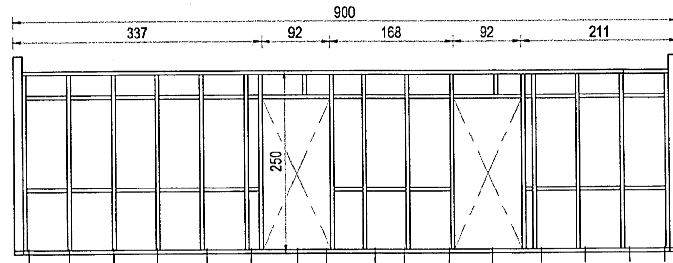
HÚS B, TIMBURGRIND NORÐUR HLIÐAR
