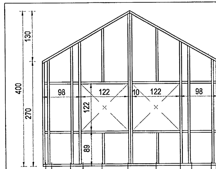
HÚS A, TIMBURGRIND AUSTUR HLIÐAR
