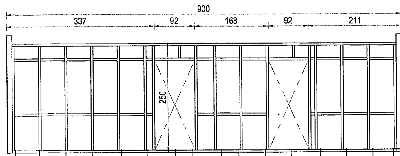
HÚS A, TIMBURGRIND SUÐUR HLIÐAR
