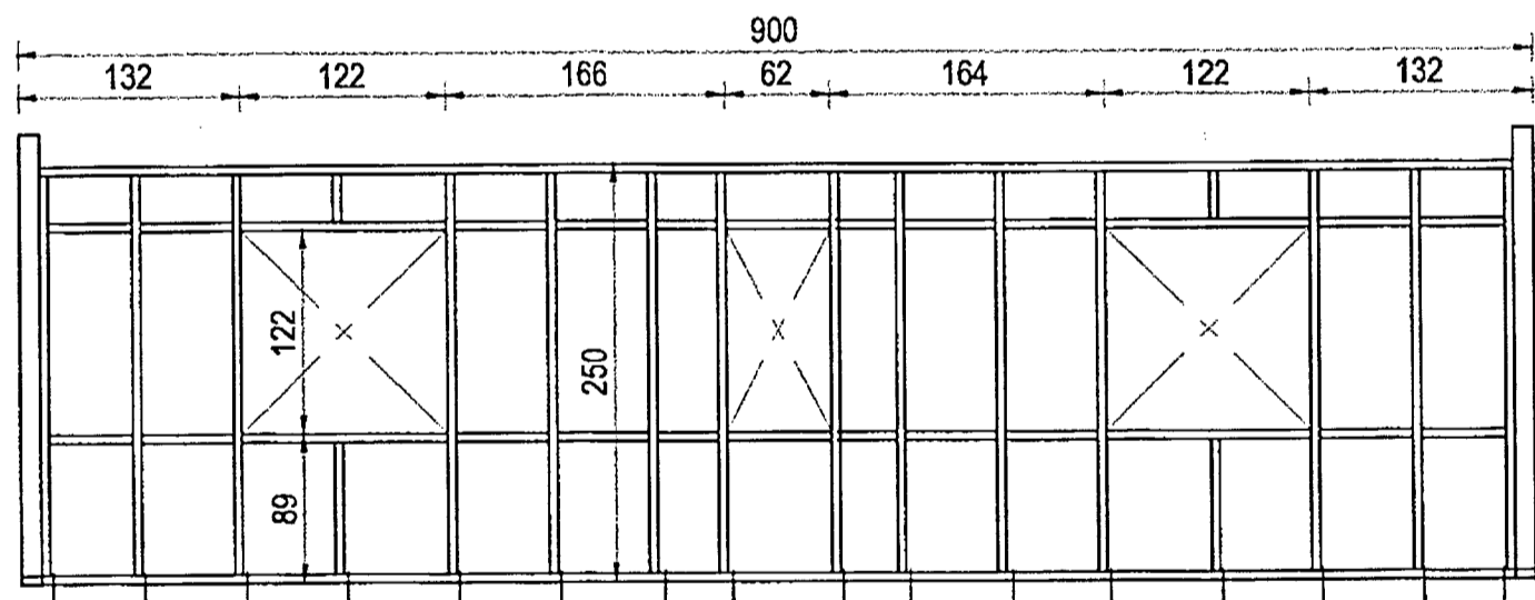
HÚS A, TIMBURGRIND NORÐUR HLIÐAR
