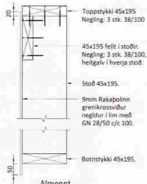
Almennt snið í grindur Mkv 1:10
