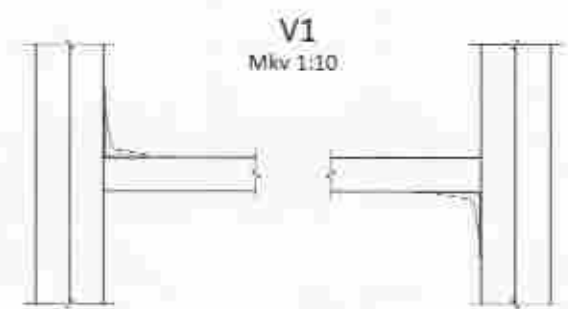
1 stk. BMF 90 vinkill m/ styrkingu Negling: 2x6 stk. KS 40/40
