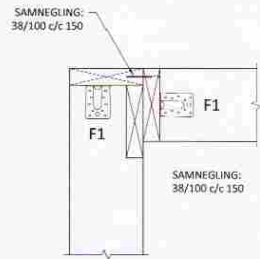
Amennur frágangur horna Mkv 1:10
