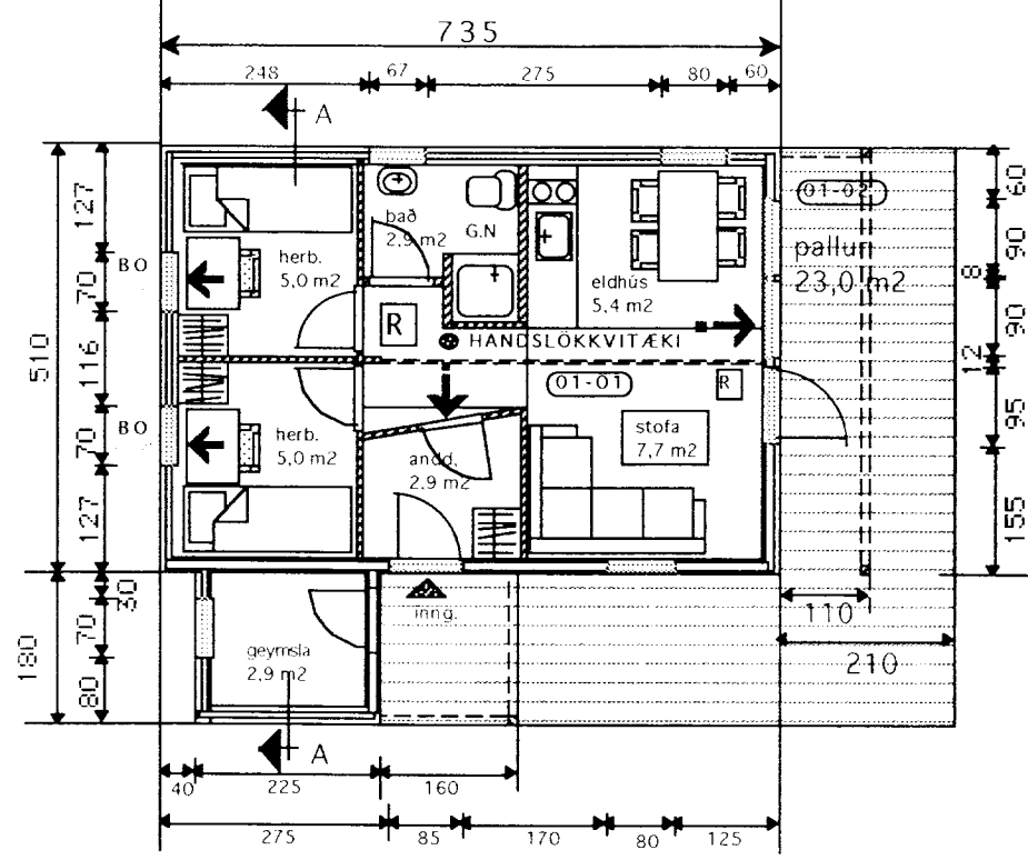
GRUNNMYND 1 :100
