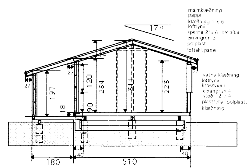
SNID A-A
