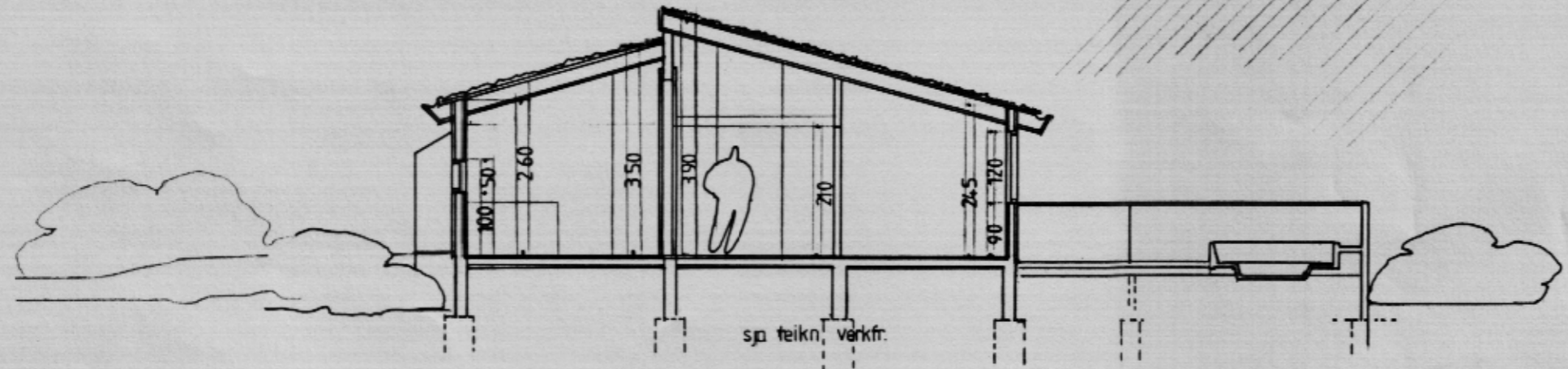
sneiðing a-a 1:100
