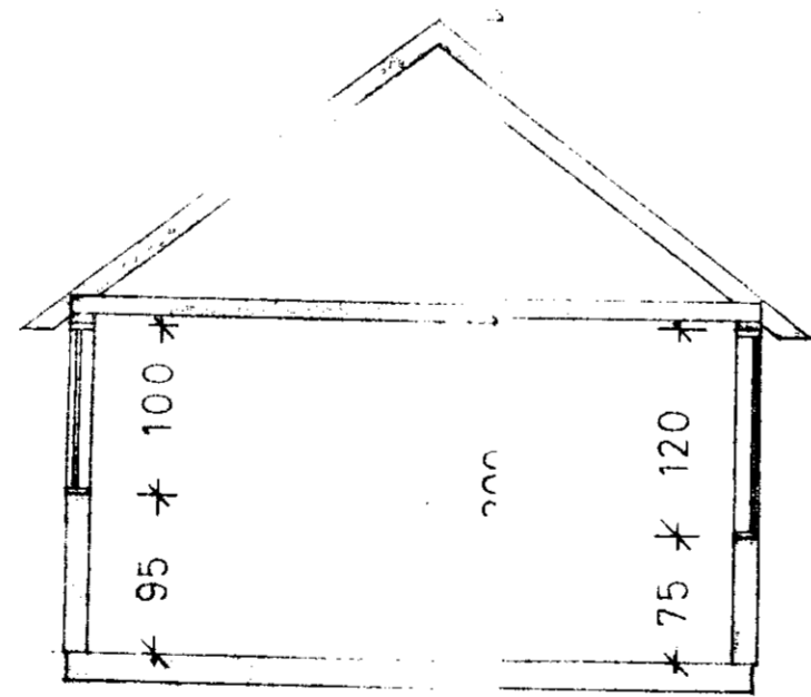
SNID A-A
