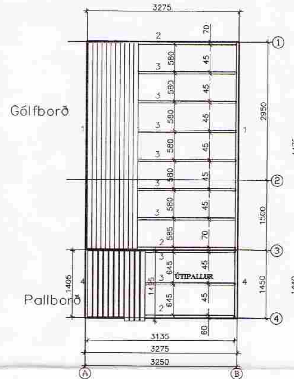
Grunnmynd gólfborð
