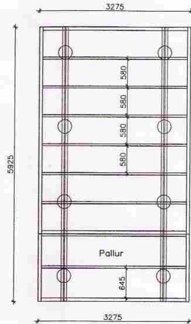
Grunnmynd dregarar
