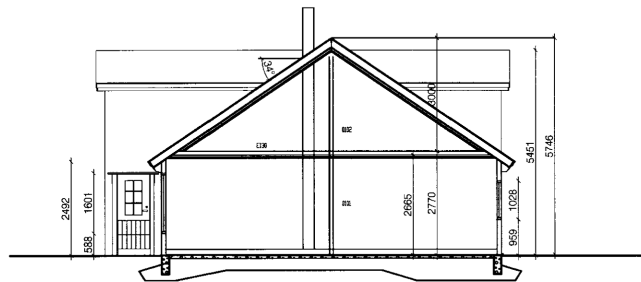
SNÍÐ A-A
