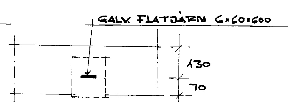
SÉRMÝND N M 1:10
