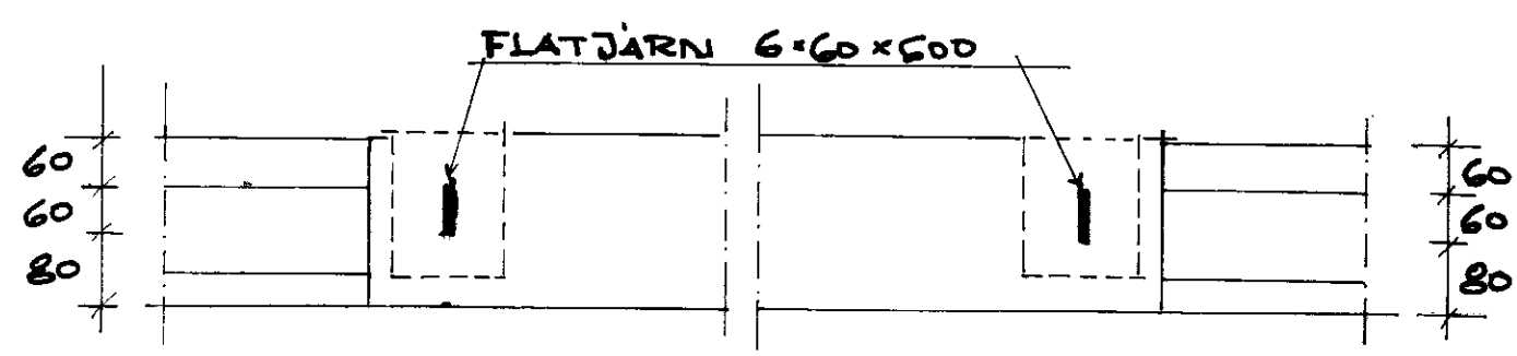
SÉRMÝND L M 1:10
