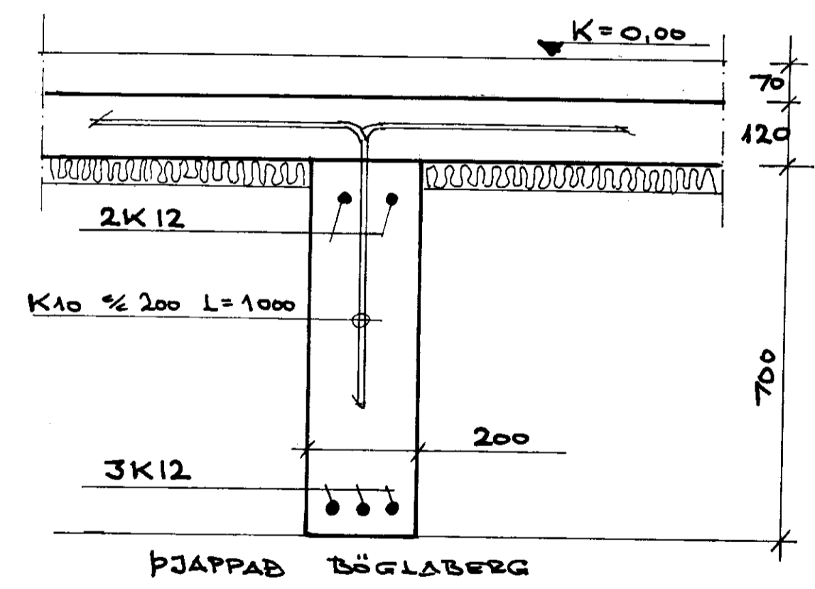
ÞJAPPAD BÖGLABERG SNIÐ E-E M 1:10
