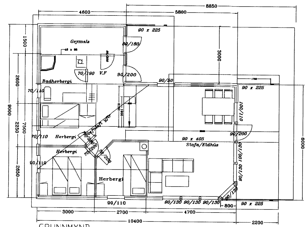
GRUNNMYND
