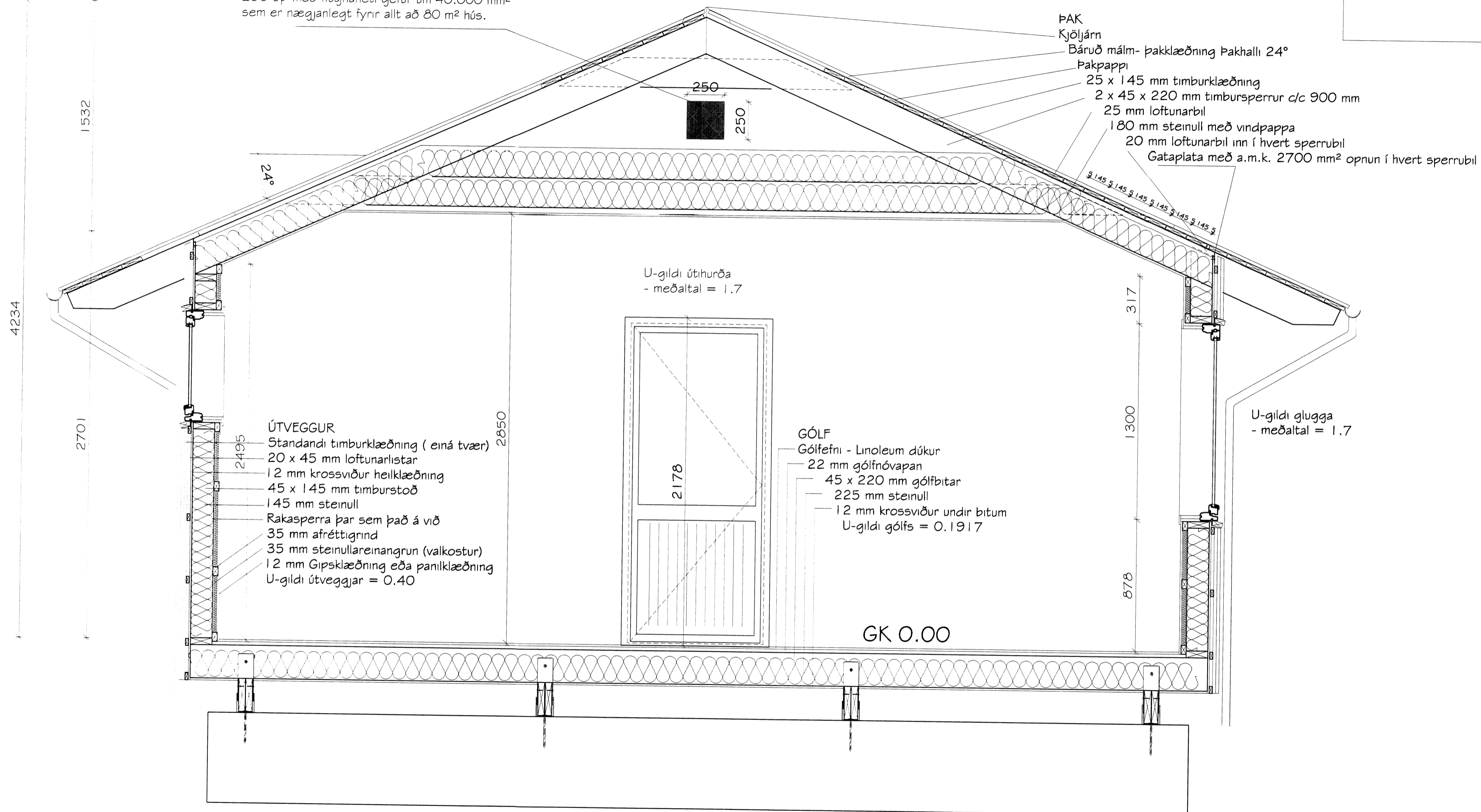
Almenn sniðmynd af rammahúsi
