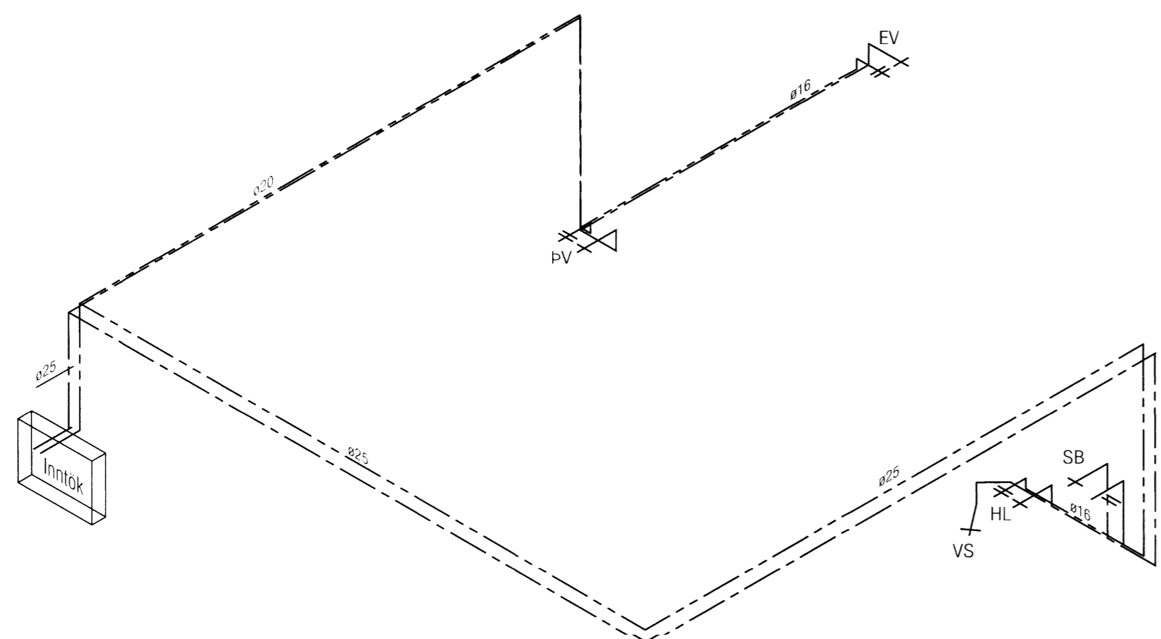
RÚMMYND VATNSLAGNA 1:50 LAGNIR ERU ÚR PEX RÖRUM (SJÁ L-01)
