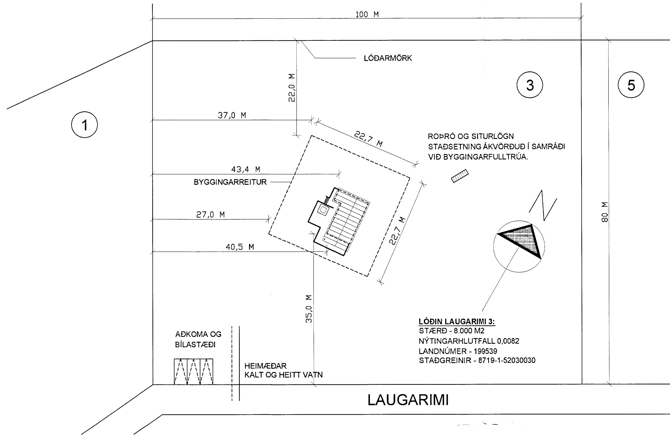
○ Afstöðumynd - 1:500
