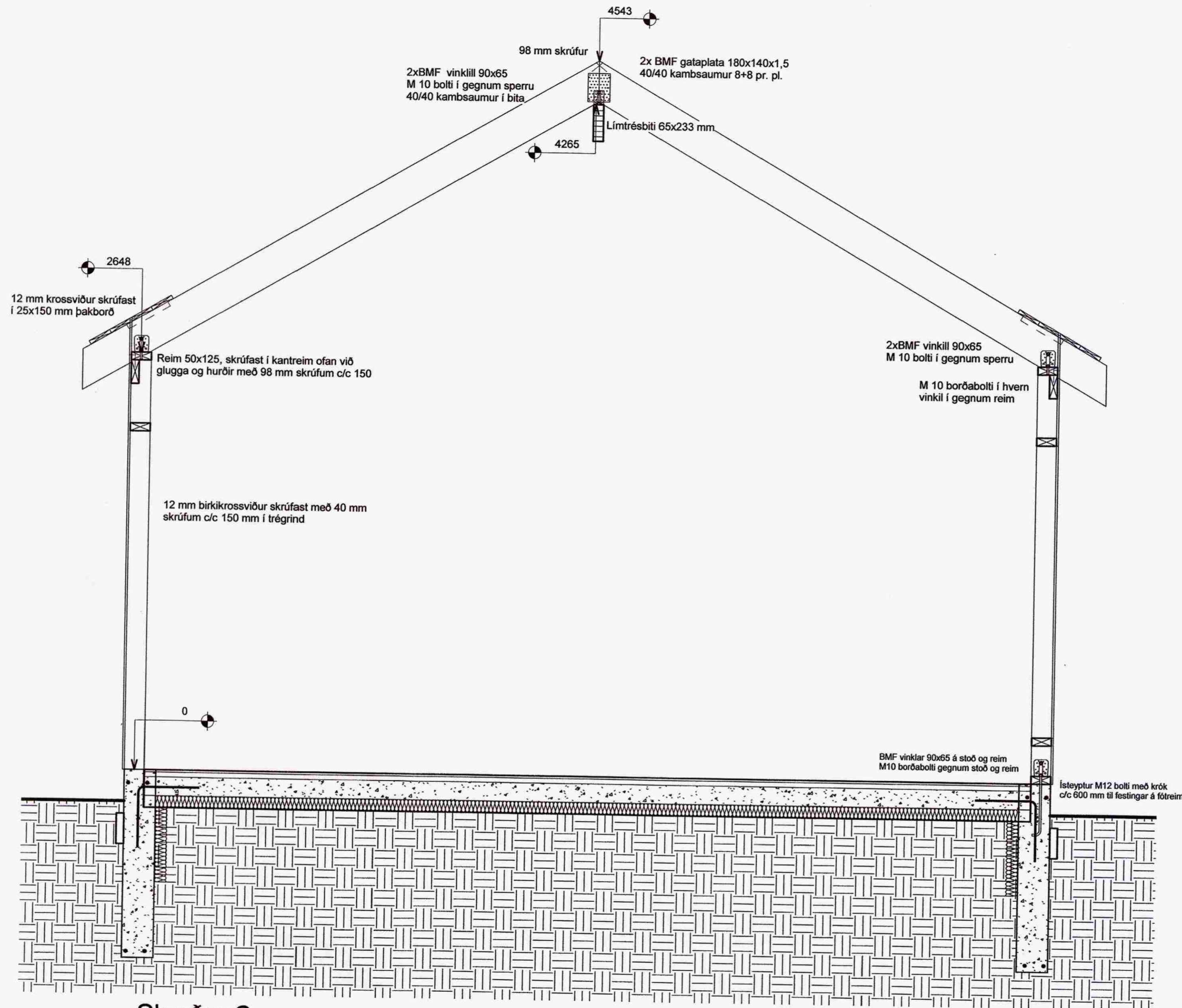
1 Skurður C 1 : 20
