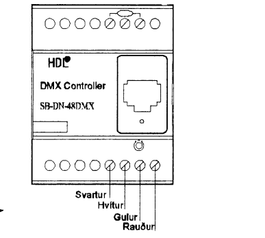
Lita tengingar á Bus kapli
