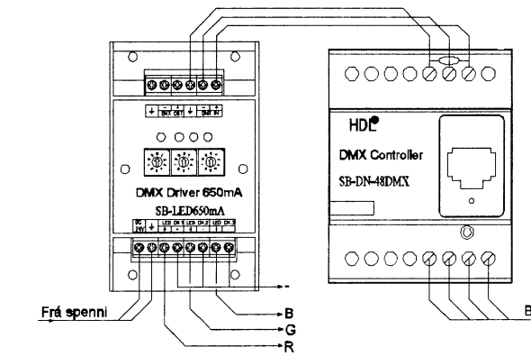
Tenging á einlita Díóðum með magnara
