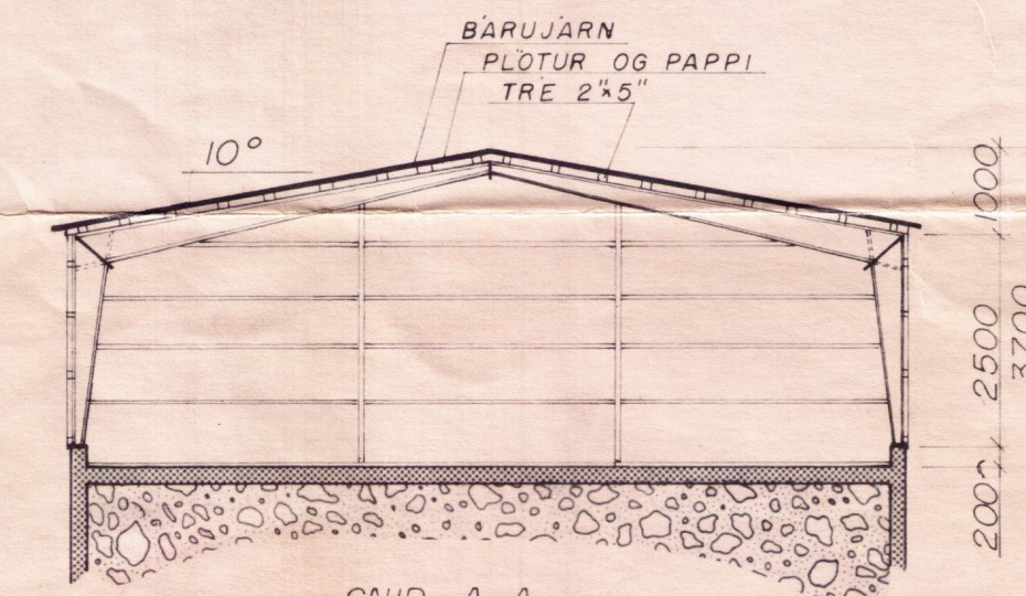
SNID A-A MKV. 1:100
