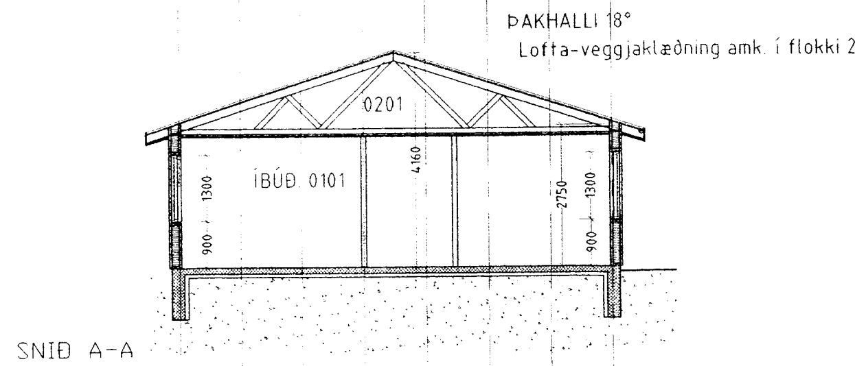
SNIÐ A-A
