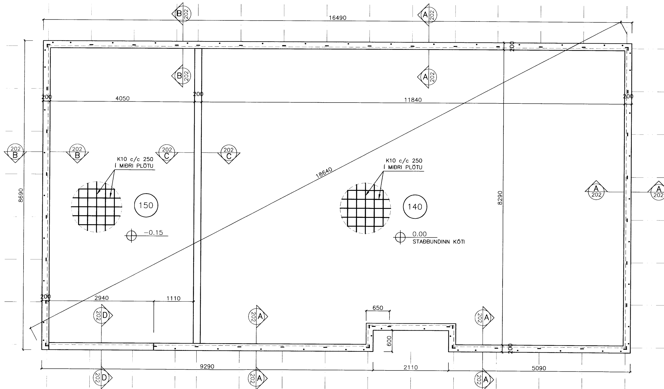
GRUNNMYND SÖKKULS Mkv. 1:50
