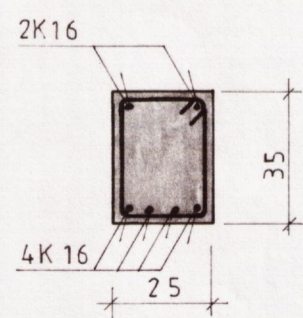
Snid A-A
