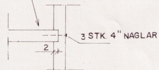
SKEYTING VIÐ GLUGGA MKV. 1:10
