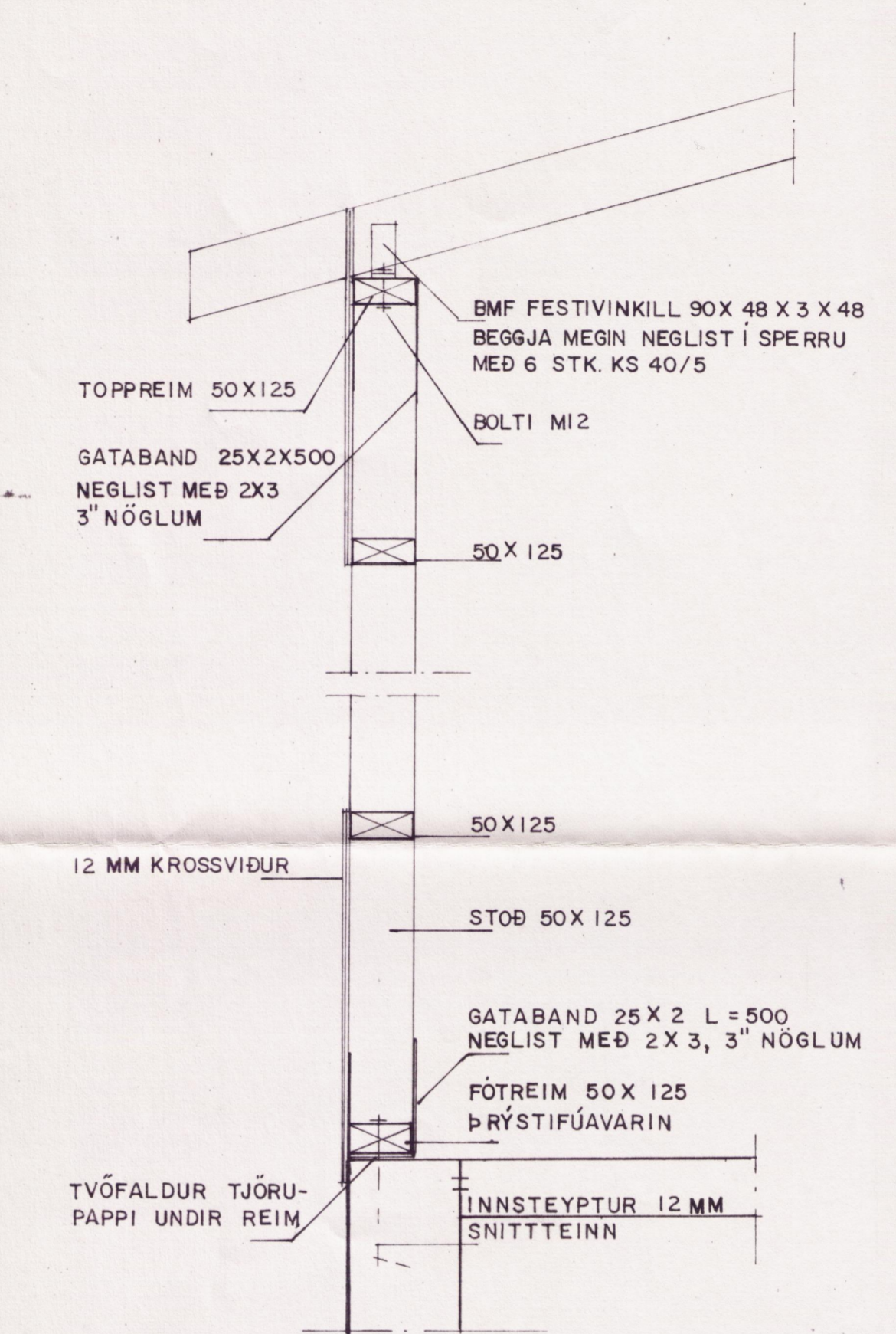
SNIÐ Í LANGVEGG MKV. 1:10
