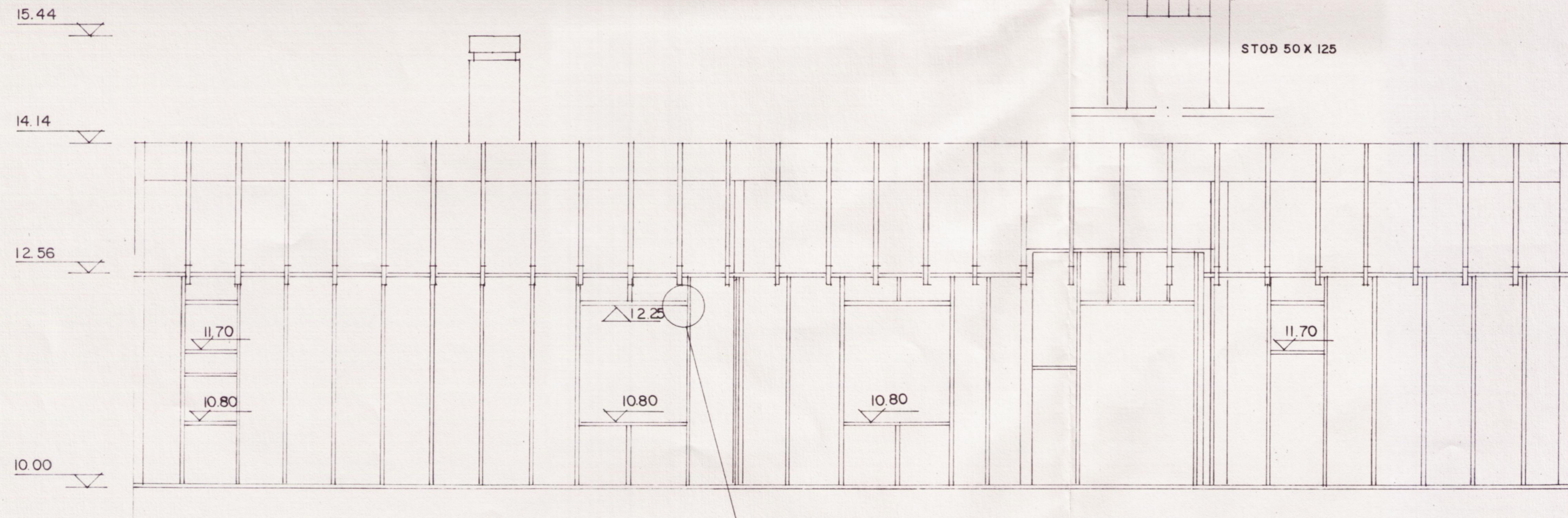
ÁSÝND NORÐUR
