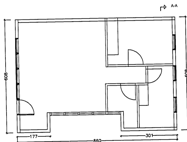
Grunnmynd mkv: 1:100
